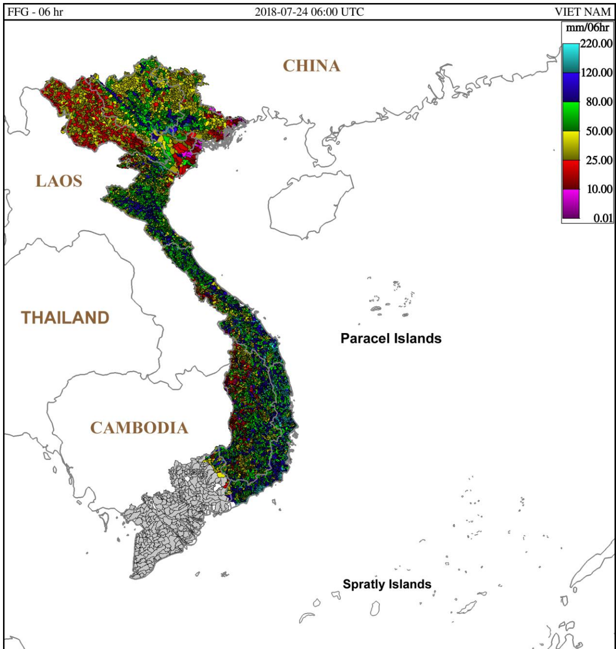
Hình 1. Ngưỡng mưa định hướng có khả năng sinh lũ quét trong 6 giờ tới tại các lưu vực từ 13h ngày 24/07/2018 giờ địa phương
