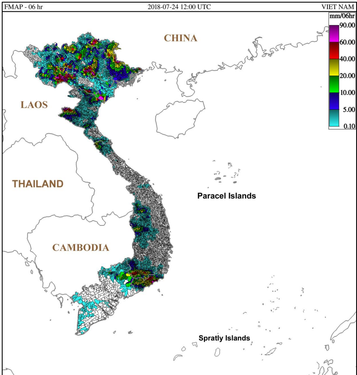
Hình 2: Dự báo lượng mưa trung bình lưu vực 6 giờ tính từ 19h ngày 24/07/2018 giờ địa phương
