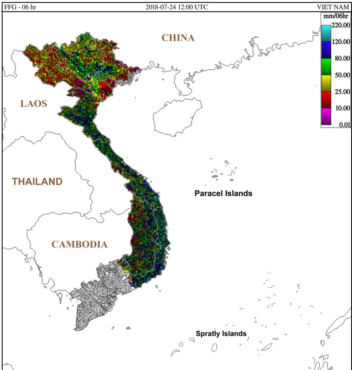
Hình 1. Ngưỡng mưa định hướng có khả năng sinh lũ quét trong 6 giờ tới tại các lưu vực từ 19h ngày 24/07/2018 giờ địa phương
