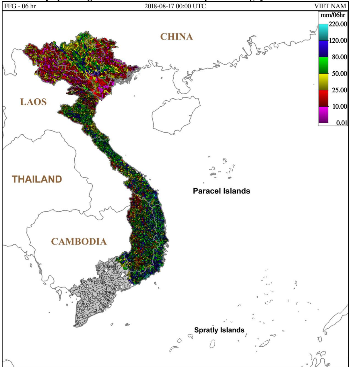
Hình 1. Ngưỡng mưa định hướng có khả năng sinh lũ quét trong 6 giờ tới tại các lưu vực từ 07h ngày 17/08/2018 giờ địa phương
