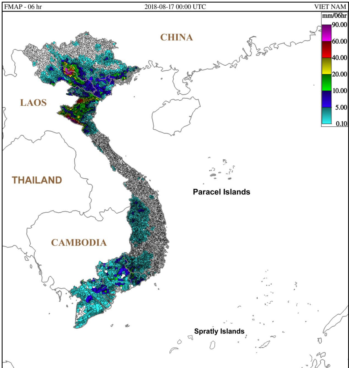
Hình 2: Dự báo lượng mưa trung bình lưu vực 6 giờ tính từ 07h ngày 17/08/2018 giờ địa phương
