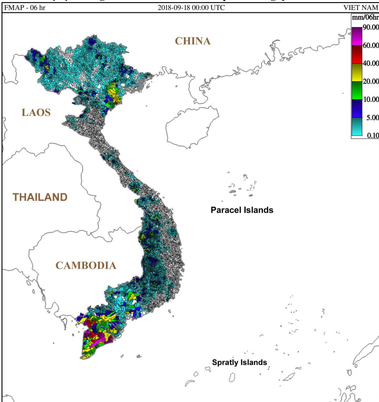
Hình 1: Dự báo lượng mưa trung bình lưu vực 6 giờ tính từ 07h ngày 18-09-2018 giờ địa phương
