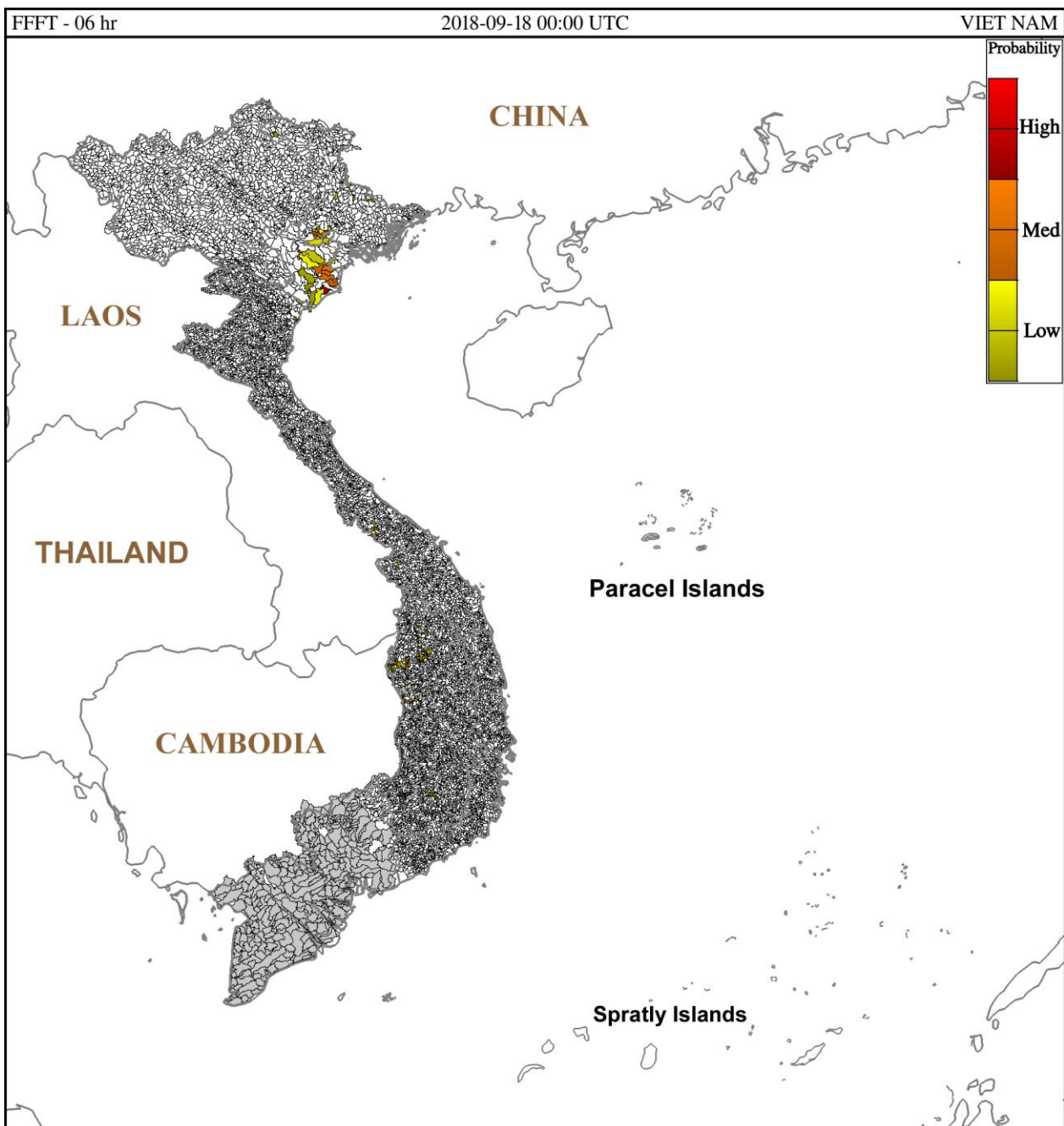
Hình 2: Nguy cơ lũ quét trong 6 giờ tới tại các lưu vực từ 07h ngày 18-09-2018 giờ địa phương
