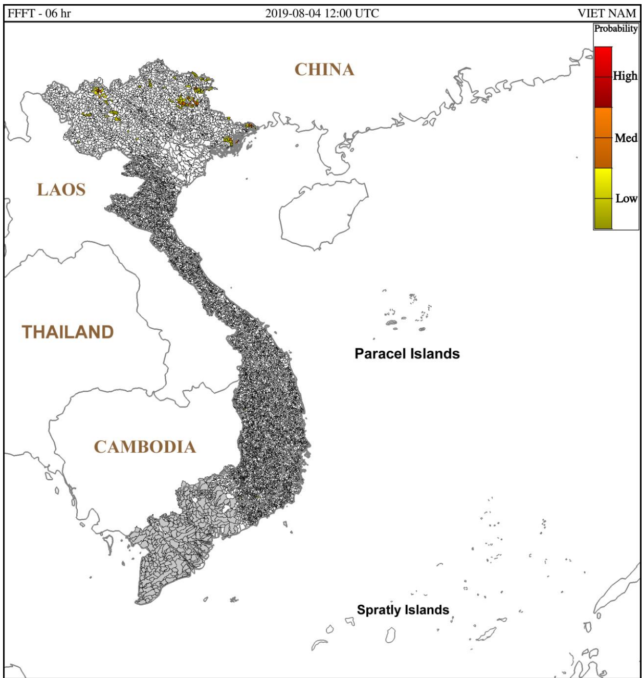
Hình 1. Nguy cơ lũ quét trong 6 giờ tới tại các lưu vực từ 19h ngày 04/08/2019 giờ địa phương
