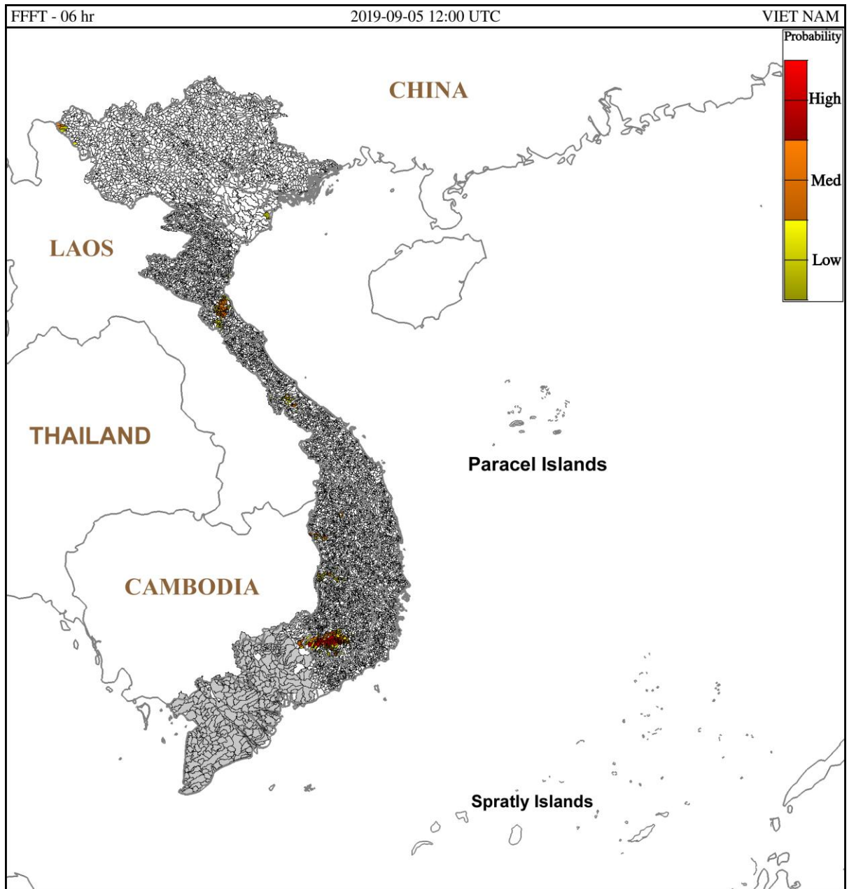
Hình 1. Nguy cơ lũ quét trong 6 giờ tới tại các lưu vực từ 19h ngày 05/9/2019 giờ địa phương
