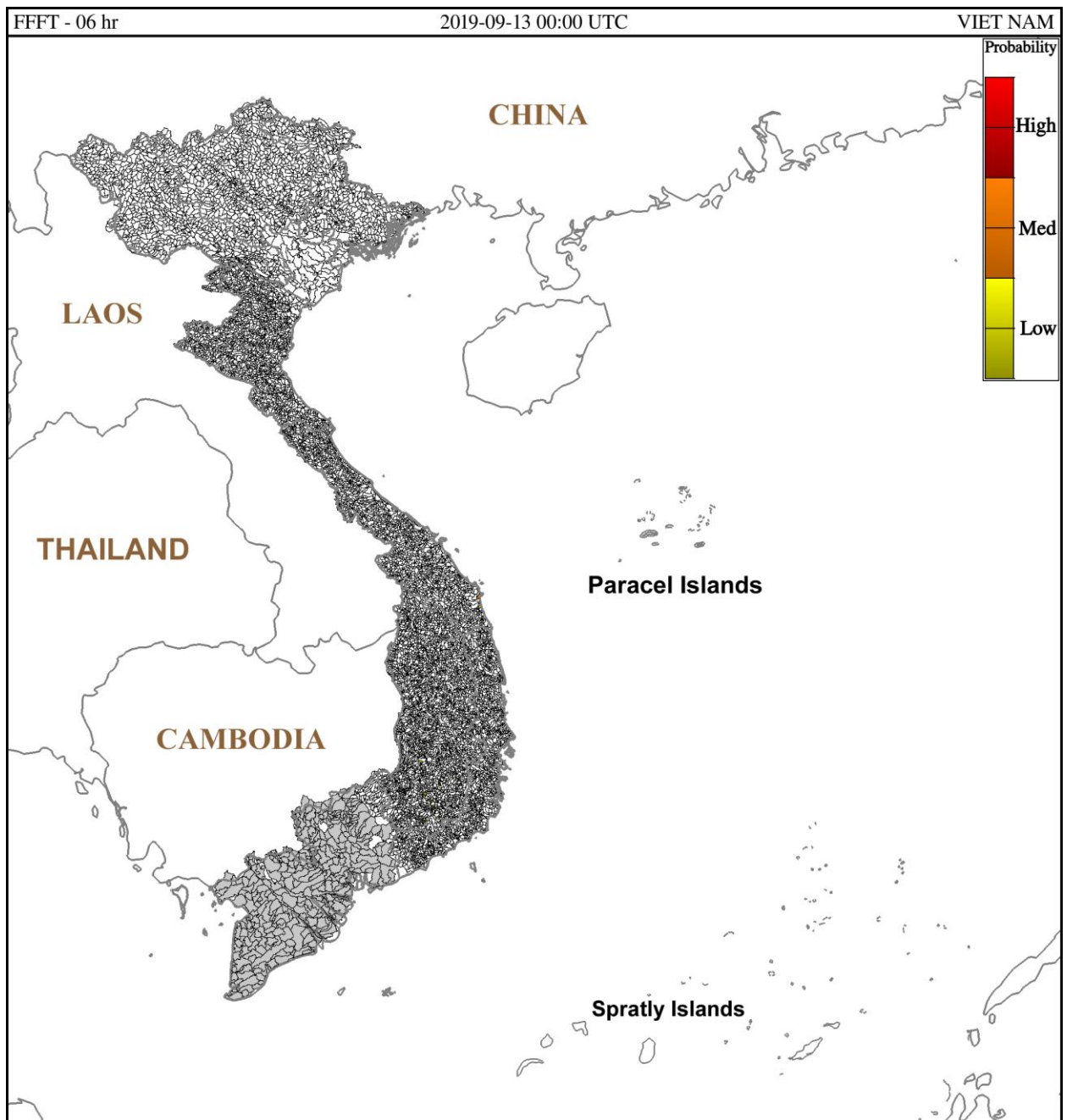
Hình 1. Nguy cơ lũ quét trong 6 giờ tới tại các lưu vực từ 07h ngày 13/9/2019 giờ địa phương
