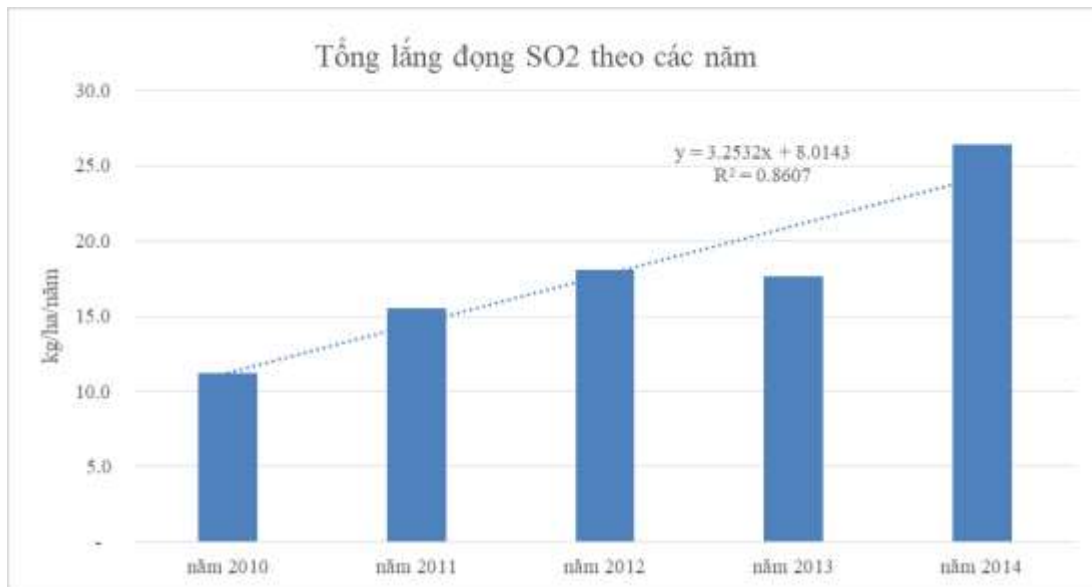
Hình 5. Tổng lắng đọng SO 2 theo các năm tại Hà Nội
