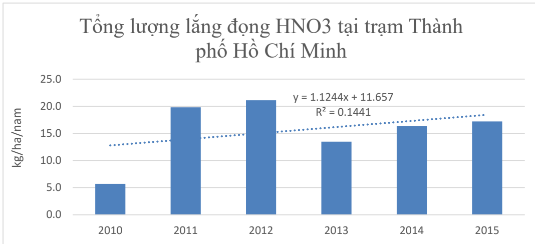
Hình 12. Tổng lắng đọng HNO 3 theo các năm tại Thành phố Hồ Chí Minh
