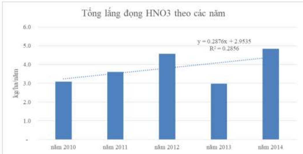
Hình 9. Tổng lắng đọng HNO 3 theo các năm tại Hòa Bình
