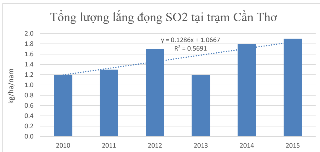
Hình 2. Tổng lắng đọng SO 2 theo các năm tại Cần Thơ
