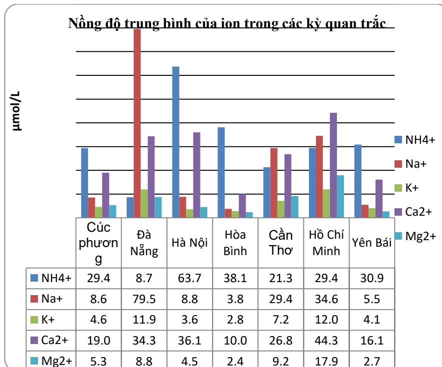
Hình 16. Nồng độ trung bình của ion trong các kỳ quan trắc
