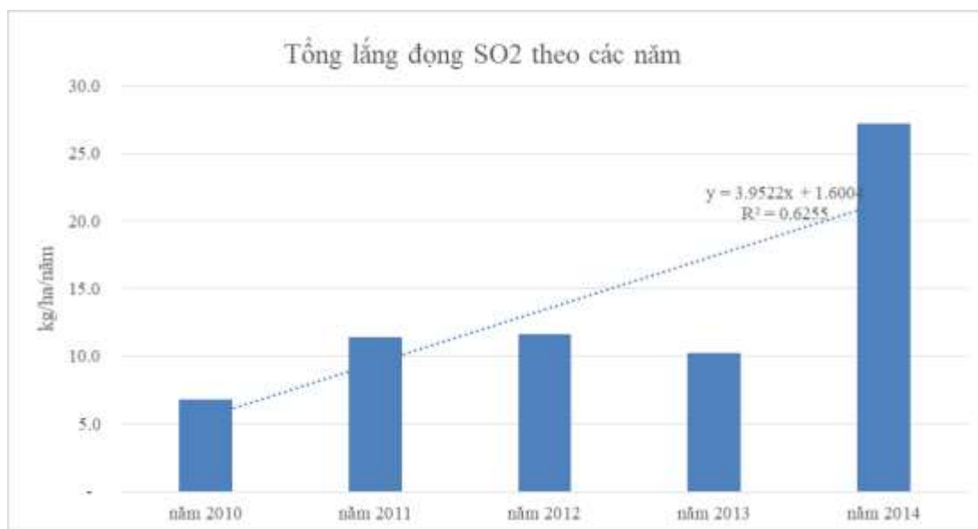
Hình 8. Tổng lắng đọng SO 2 theo các năm tại Hòa Bình
