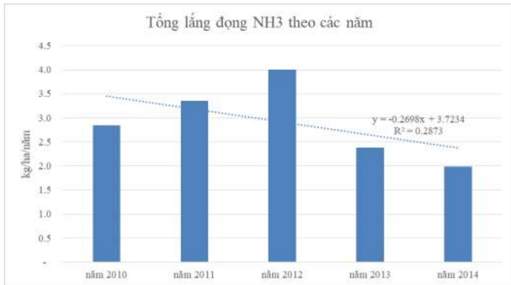
Hình 10. Tổng lắng đọng NH 3 theo các năm tại Hòa Bình
