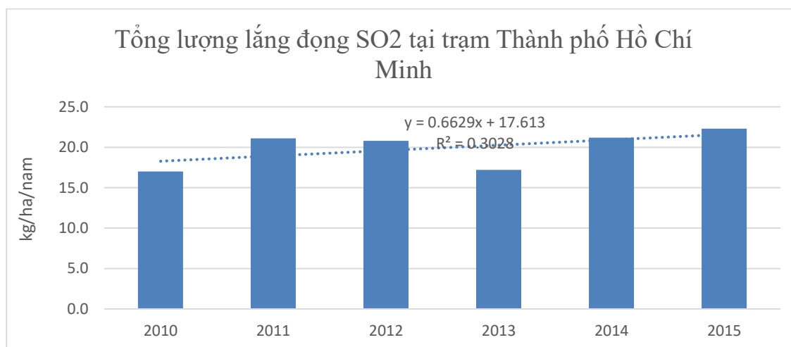
Hình 11. Tổng lắng đọng SO 2 theo các năm tại Thành phố Hồ Chí Minh
