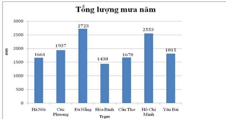
Hình 14. Tổng lượng mưa năm 2016
