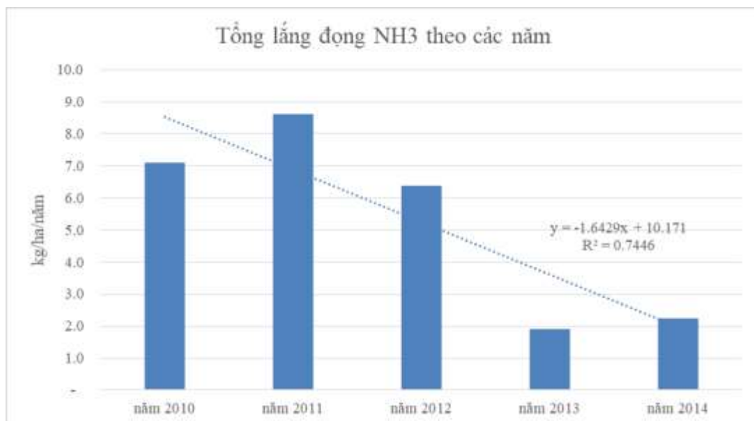
Hình 7. Tổng lắng đọng NH 3 theo các năm tại Hà Nội
