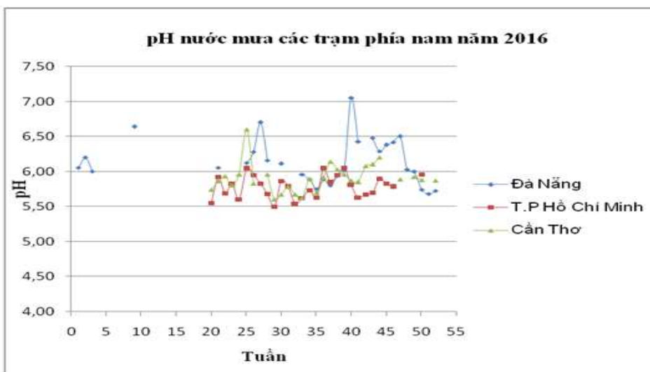
Hình 15. PH nước mưa các trạm năm 2016
