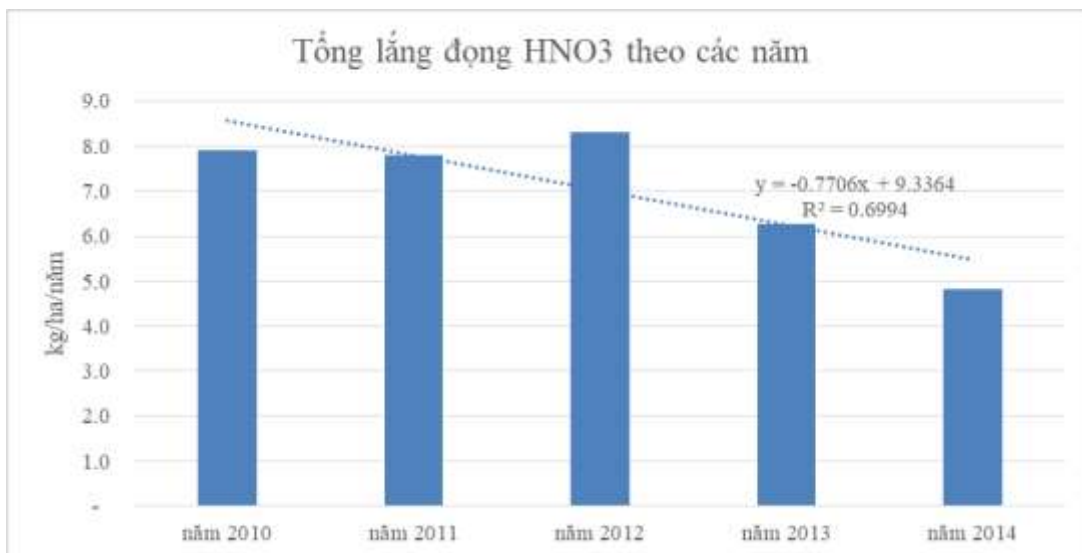
Hình 6. Tổng lắng đọng HNO 3 theo các năm tại Hà Nội
