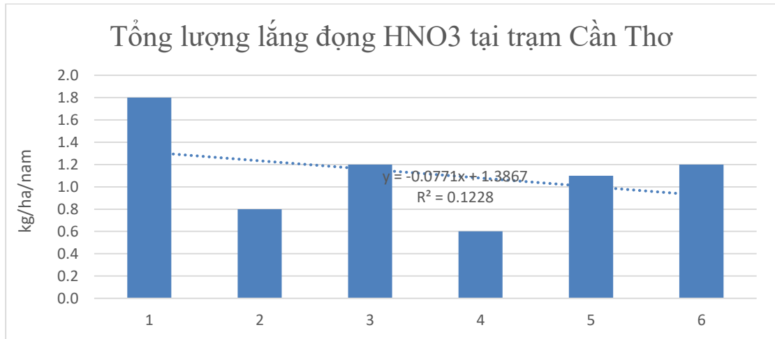
Hình 3. Tổng lắng đọng HNO 3 theo các năm tại Cần Thơ
