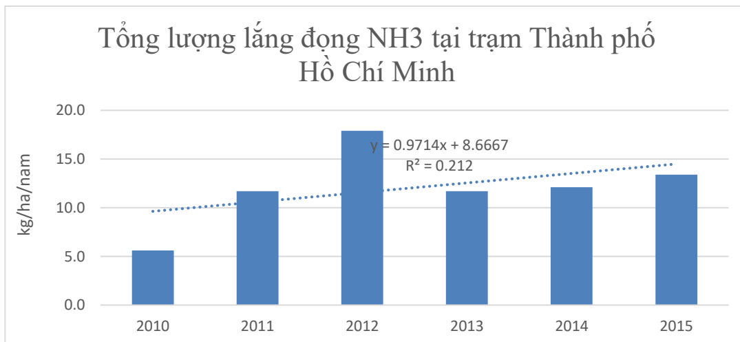
Hình 13. Tổng lắng đọng NH 3 theo các năm tại Thành phố Hồ Chí Minh
