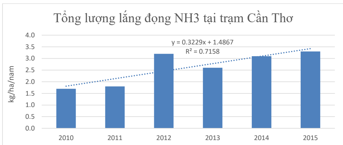
Hình 4. Tổng lắng đọng NH 3 theo các năm tại Cần Thơ
