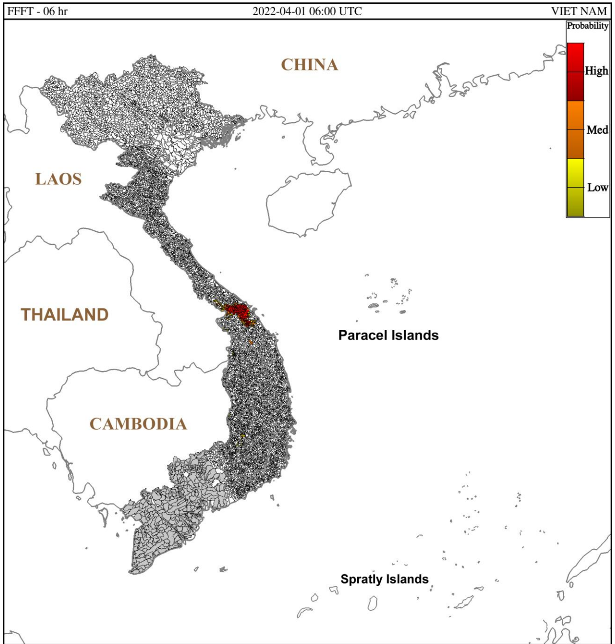
Hình 1. Nguy cơ lũ quét trong 6 giờ tới tại các lưu vực từ 13h ngày 01/04/2022 giờ địa phương
