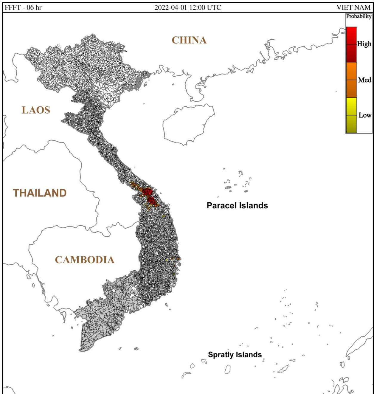
Hình 1. Nguy cơ lũ quét trong 6 giờ tới tại các lưu vực từ 19h ngày 01/04/2022 giờ địa phương
