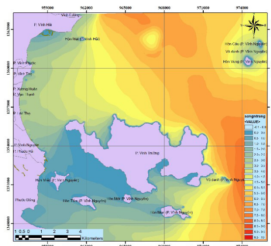
Hình 20. Phân bố sóng do bão Damrey khu vực vịnh Nha Trang
