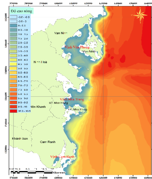
Hình 19. Phân bố sóng do bão Damrey khu vực biển Khánh Hòa
