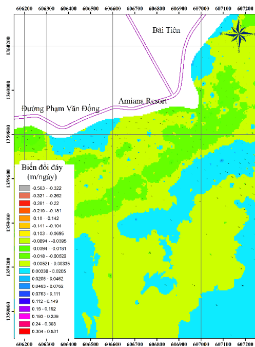
Hình 27. Xói lở khu vực Bãi Tiên
