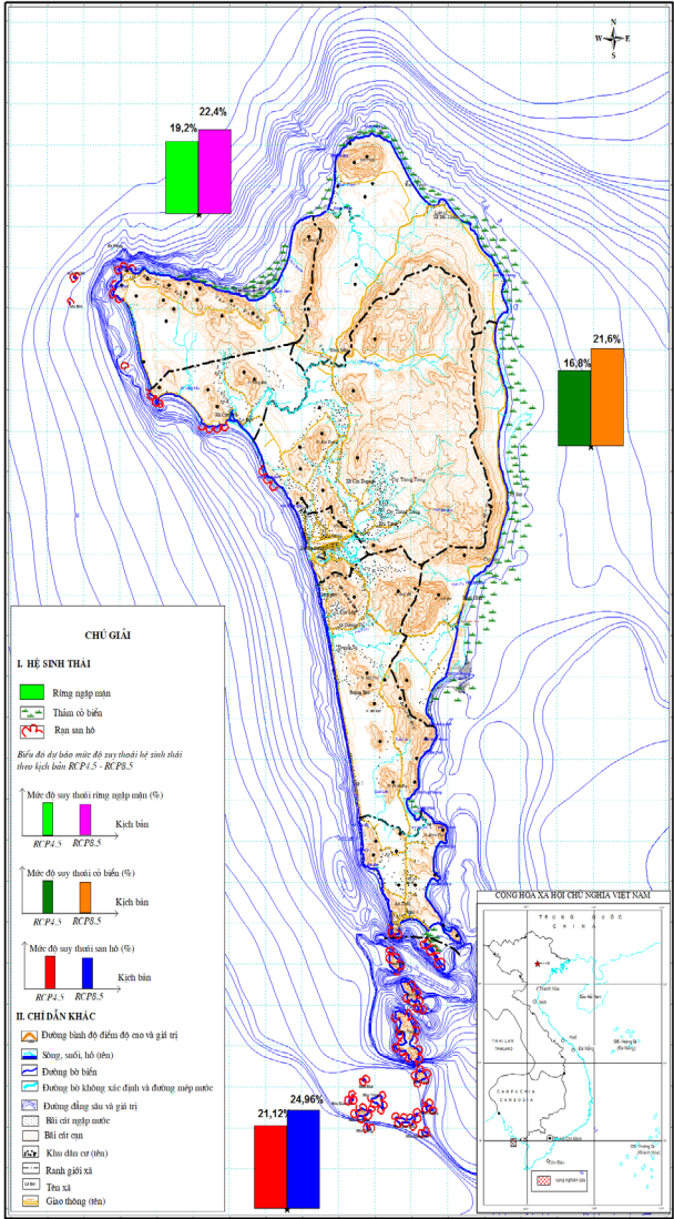
Hình 2. Sơ đồ dự báo mức độ suy thoái các hệ sinh thái biển Phú Quốc theo kịch bản BĐKH NBD RCP4.5 và RCP8.5 cho năm 2050
