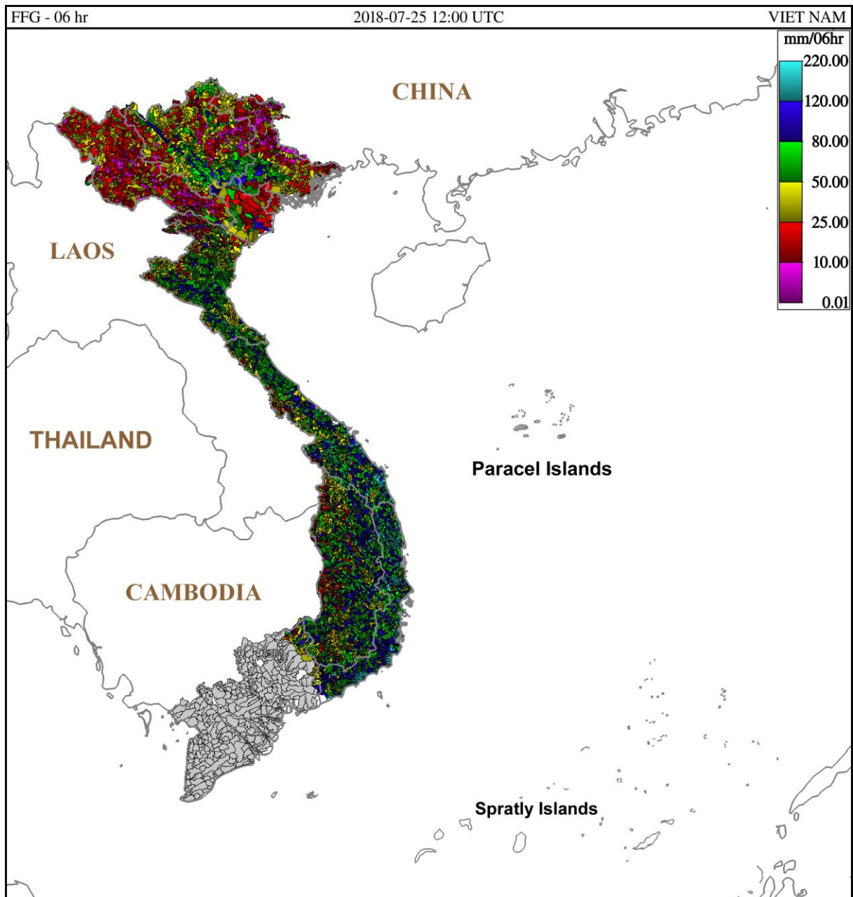
Hình 1. Ngưỡng mưa định hướng có khả năng sinh lũ quét trong 6 giờ tới tại các lưu vực từ 19h ngày 25/07/2018 giờ địa phương
