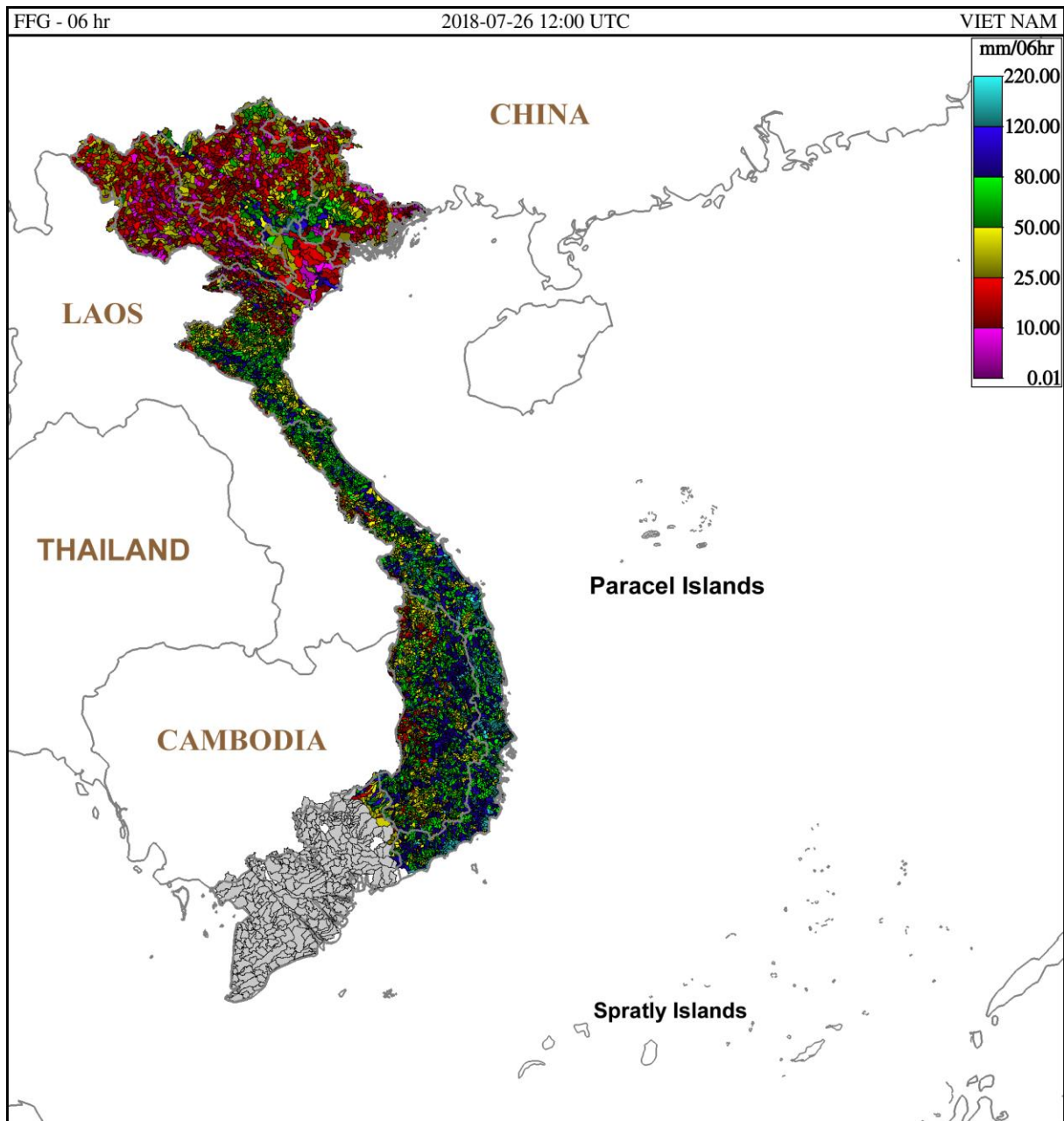
Hình 1. Ngưỡng mưa định hướng có khả năng sinh lũ quét trong 6 giờ tới tại các lưu vực từ 19h ngày 26/07/2018 giờ địa phương
