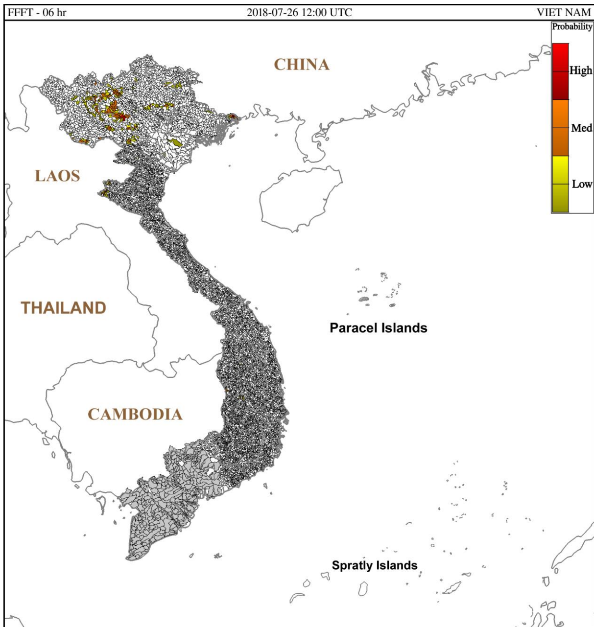
Hình 3: Nguy cơ lũ quét trong 6 giờ tới tại các lưu vực từ 19h ngày 26/07/2018 giờ địa phương
