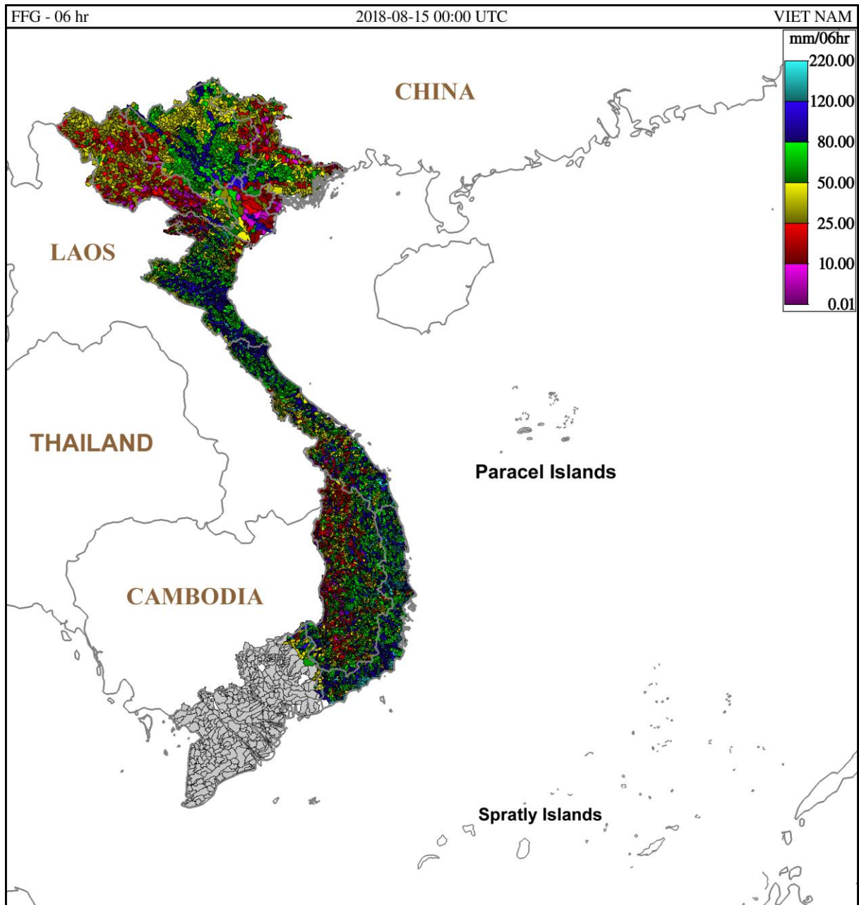
Hình 1. Ngưỡng mưa định hướng có khả năng sinh lũ quét trong 6 giờ tới tại các lưu vực từ 07h ngày 15/8/2018 giờ địa phương
