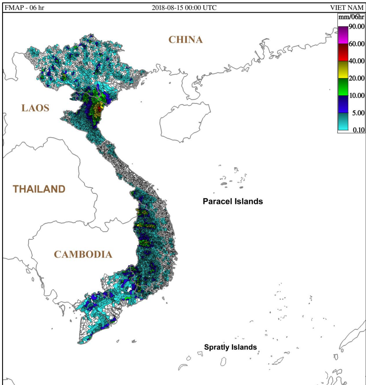
Hình 2: Dự báo lượng mưa trung bình lưu vực 6 giờ tính từ 07h ngày 15/8/2018 giờ địa phương
