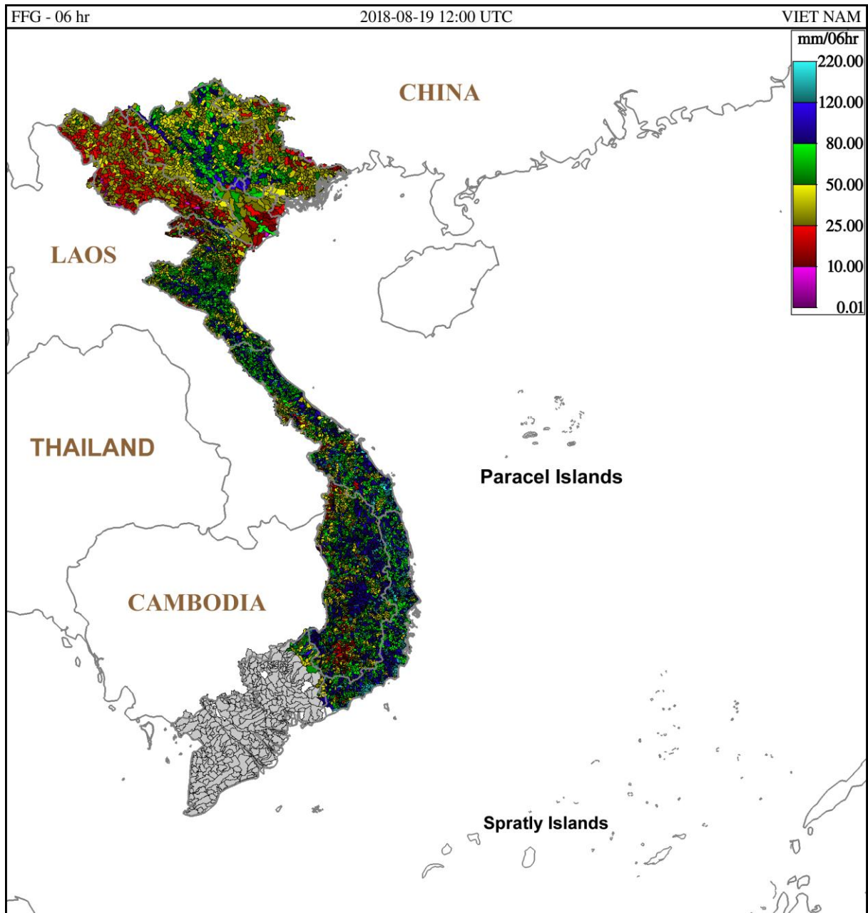
Hình 1. Ngưỡng mưa định hướng có khả năng sinh lũ quét trong 6 giờ tới tại các lưu vực từ 19h ngày 19/08/2018 giờ địa phương
