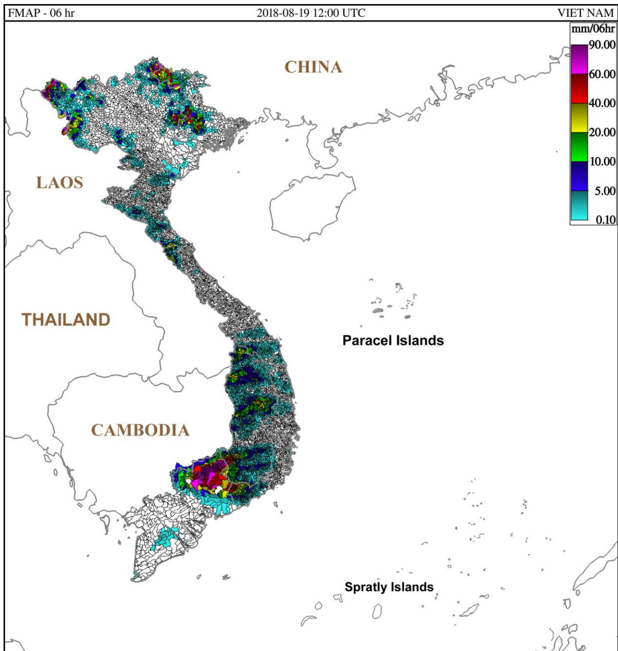
Hình 2: Dự báo lượng mưa trung bình lưu vực 6 giờ tính từ 19h ngày 19/08/2018 giờ địa phương
