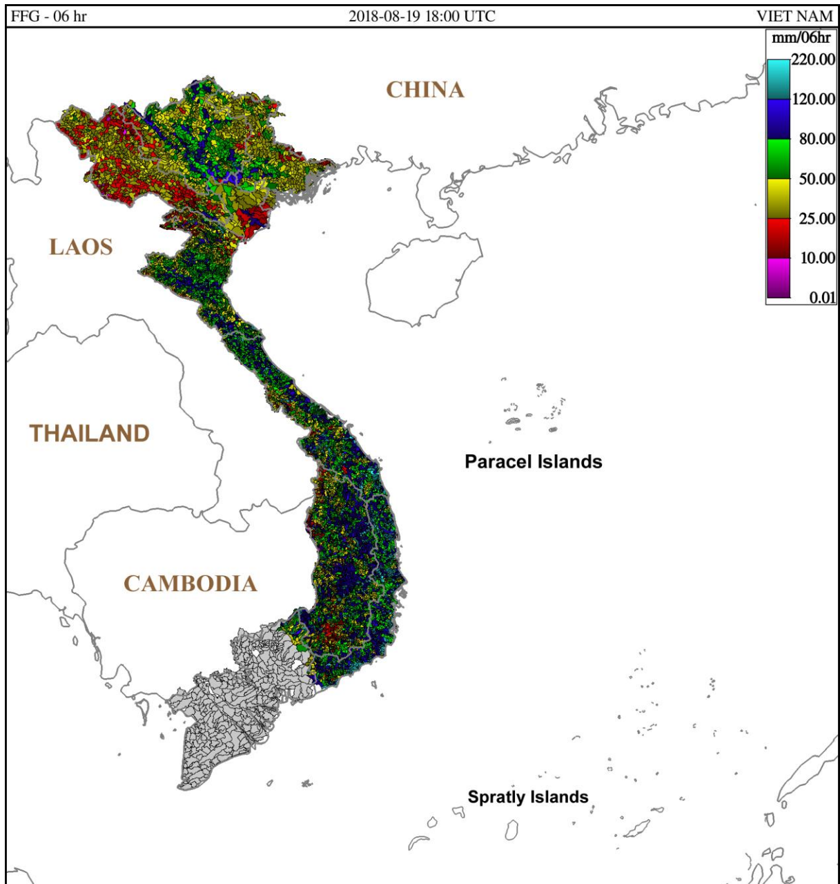
Hình 1. Ngưỡng mưa định hướng có khả năng sinh lũ quét trong 6 giờ tới tại các lưu vực từ 01h ngày 20/08/2018 giờ địa phương
