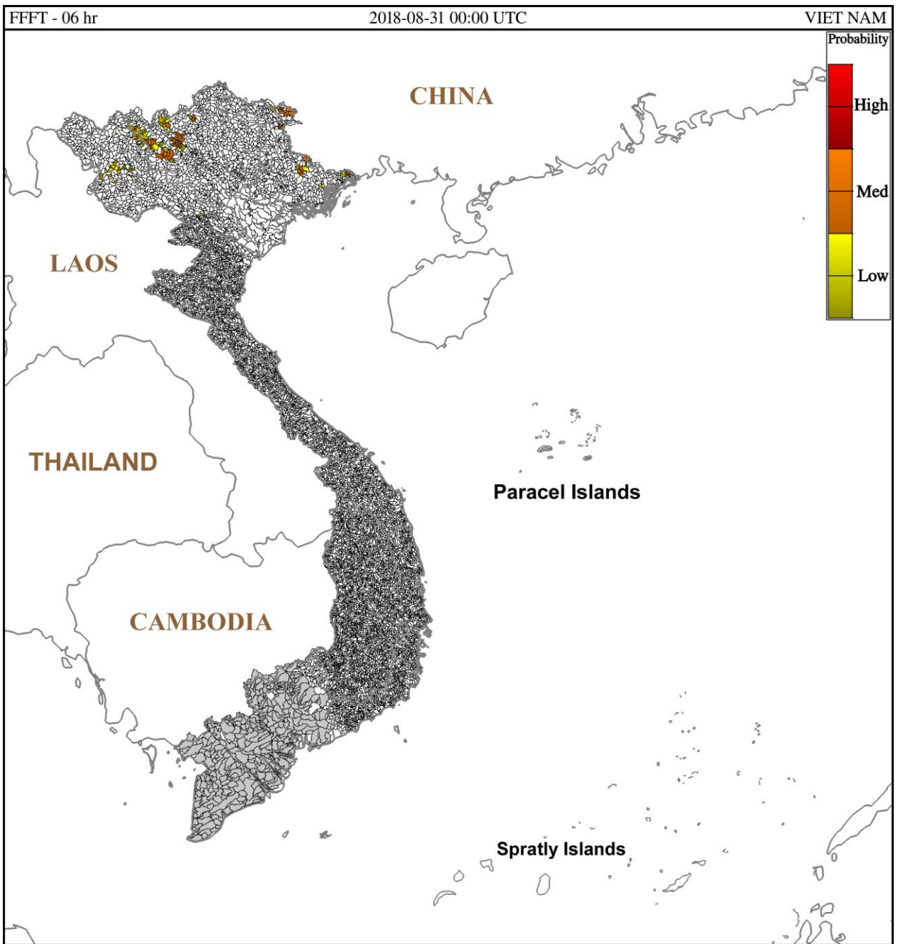
Hình 2: Nguy cơ lũ quét trong 6 giờ tới tại các lưu vực từ 07h ngày 31-08-2018 giờ địa phương
