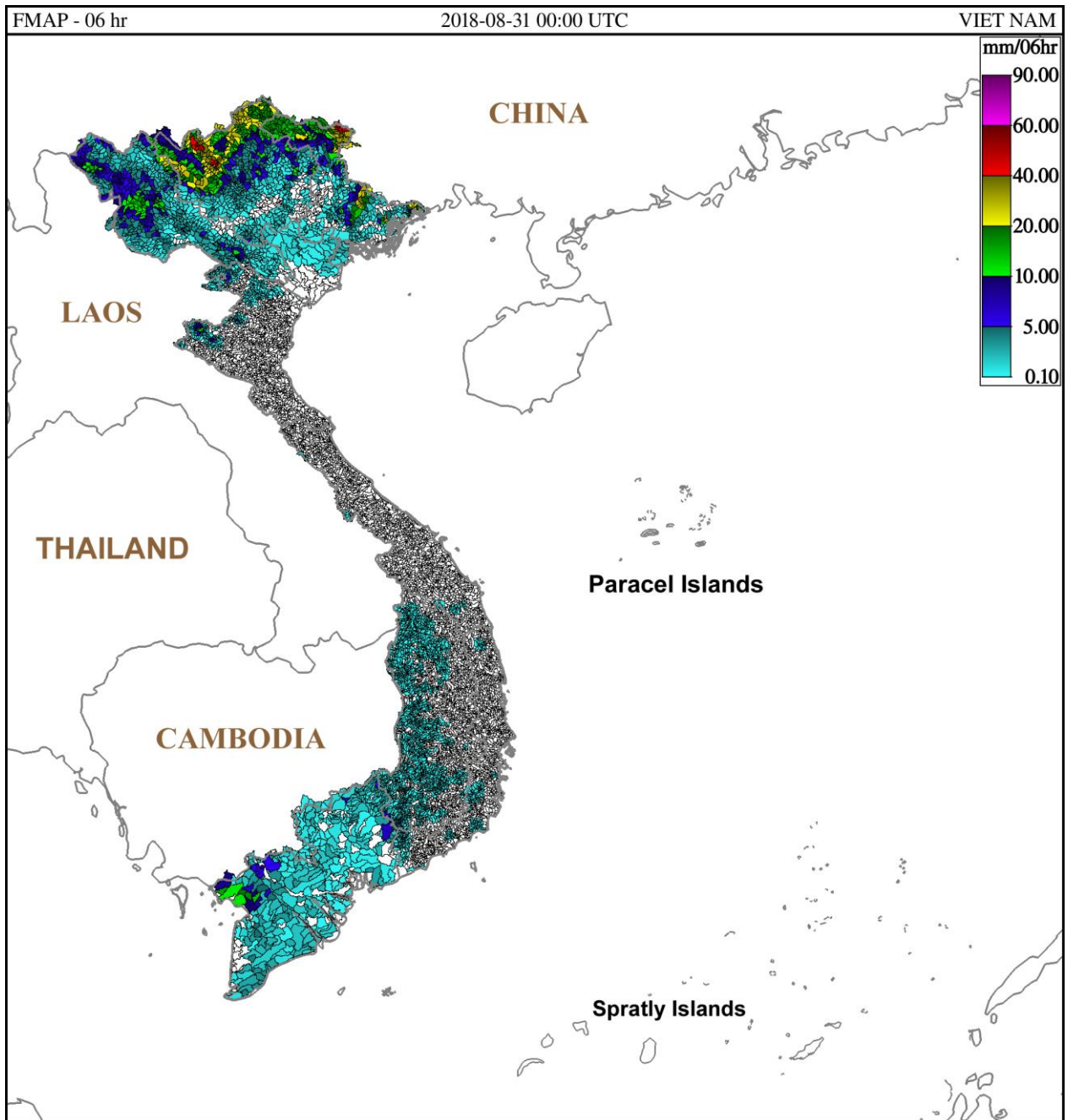
Hình 1: Dự báo lượng mưa trung bình lưu vực 6 giờ tính từ 07h ngày 31-08-2018 giờ địa phương
