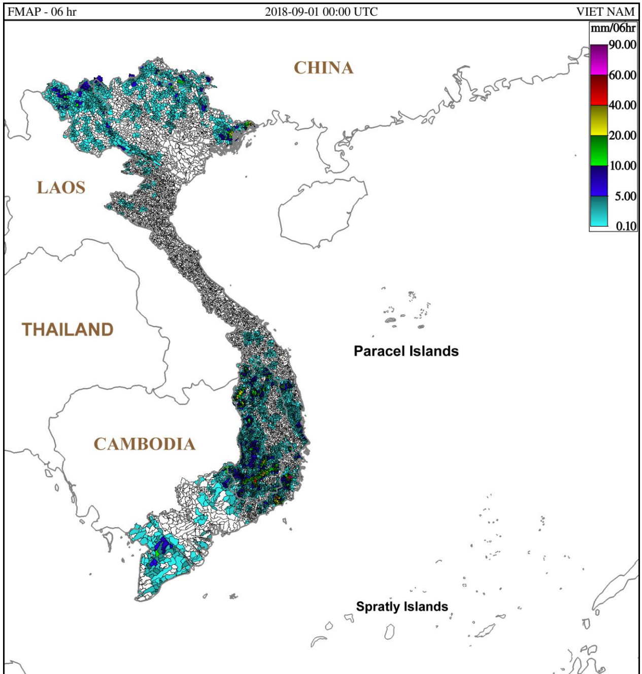
Hình 1: Dự báo lượng mưa trung bình lưu vực 6 giờ tính từ 07h ngày 01-09-2018 giờ địa phương
