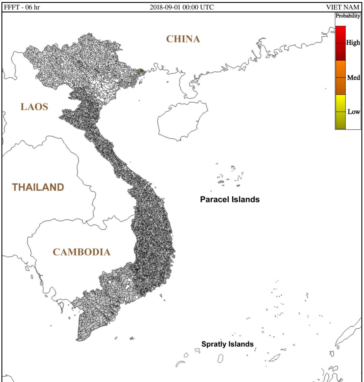
Hình 2: Nguy cơ lũ quét trong 6 giờ tới tại các lưu vực từ 07h ngày 01-09-2018 giờ địa phương
