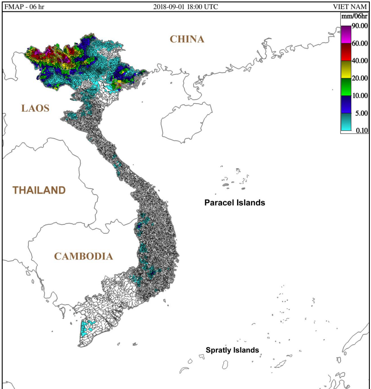
Hình 1: Dự báo lượng mưa trung bình lưu vực 6 giờ tính từ 01h ngày 02-09-2018 giờ địa phương
