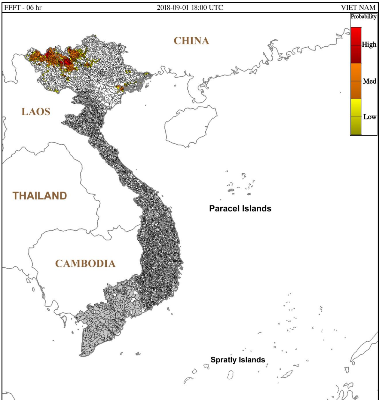
Hình 2: Nguy cơ lũ quét trong 6 giờ tới tại các lưu vực từ 01h ngày 02-09-2018 giờ địa phương
