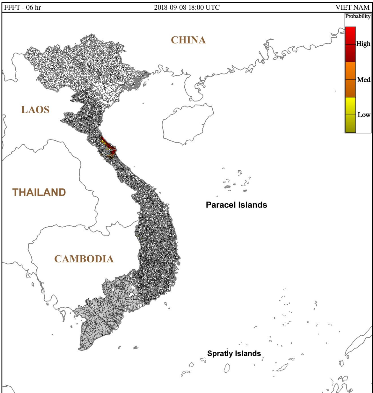
Hình 2: Nguy cơ lũ quét trong 6 giờ tới tại các lưu vực từ 01h ngày 09-9-2018 giờ địa phương
