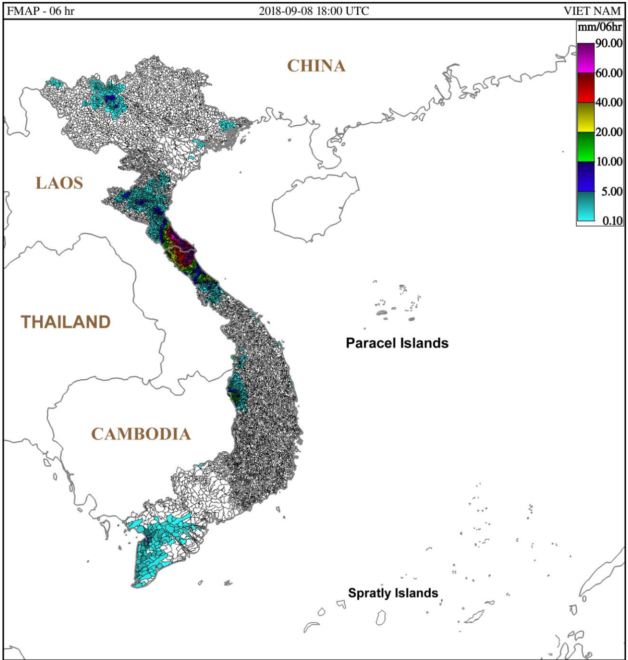
Hình 1: Dự báo lượng mưa trung bình lưu vực 6 giờ tính từ 01h ngày 09-09-2018 giờ địa phương
