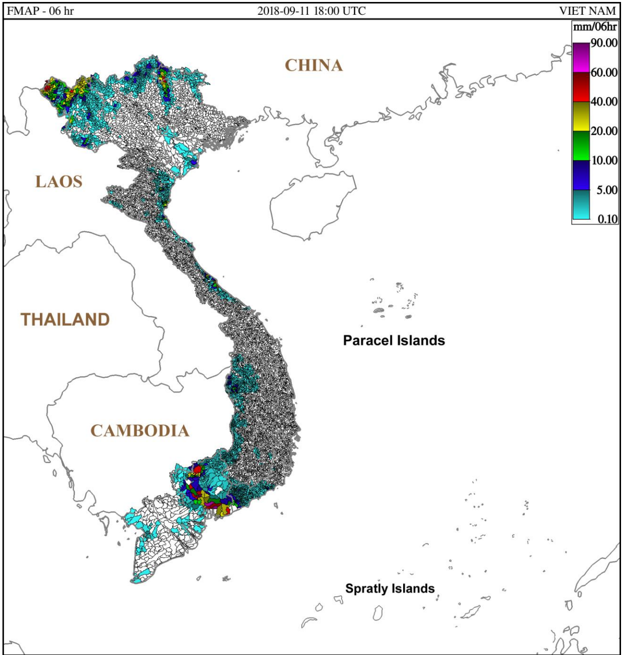
Hình 1: Dự báo lượng mưa trung bình lưu vực 6 giờ tính từ 01h ngày 12-09-2018 giờ địa phương
