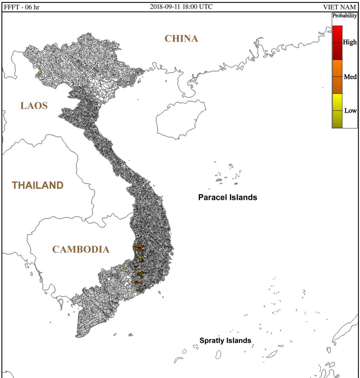
Hình 2: Nguy cơ lũ quét trong 6 giờ tới tại các lưu vực từ 01h ngày 12-9-2018 giờ địa phương
