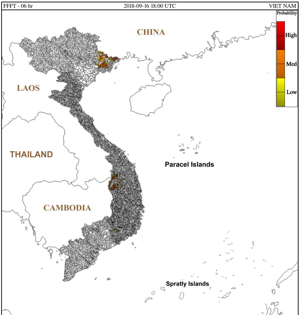
Hình 2: Nguy cơ lũ quét trong 6 giờ tới tại các lưu vực từ 01h ngày 17-9-2018 giờ địa phương
