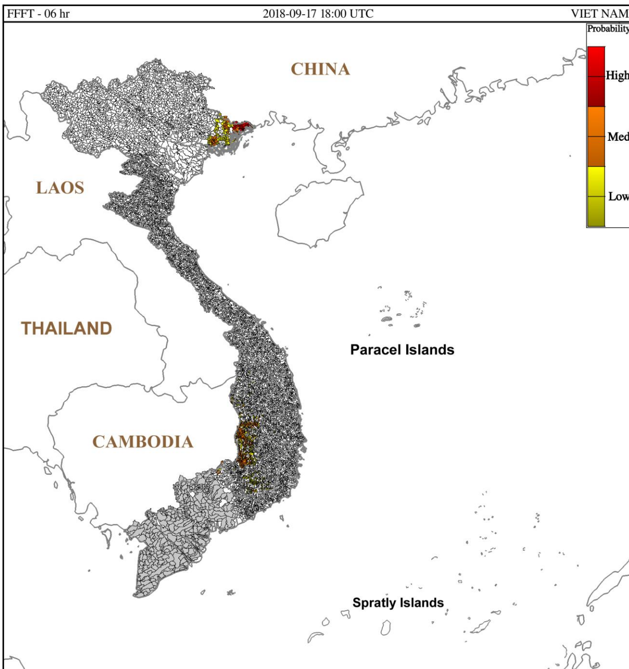
Hình 2: Nguy cơ lũ quét trong 6 giờ tới tại các lưu vực từ 01h ngày 18-09-2018 giờ địa phương
