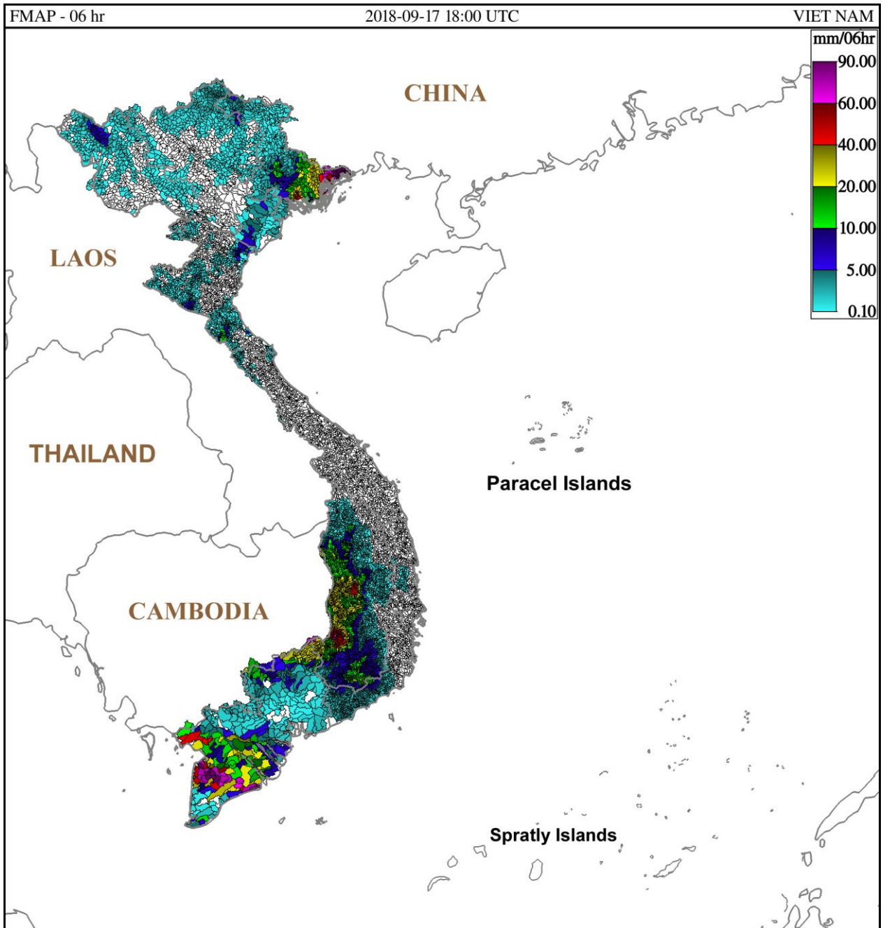
Hình 1: Dự báo lượng mưa trung bình lưu vực 6 giờ tính từ 01h ngày 18-09-2018 giờ địa phương
