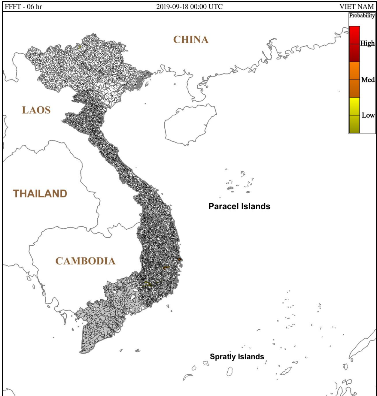
Hình 1: Nguy cơ lũ quét trong 6 giờ tới tại các lưu vực từ 7h ngày 18/09/2019 giờ địa phương
