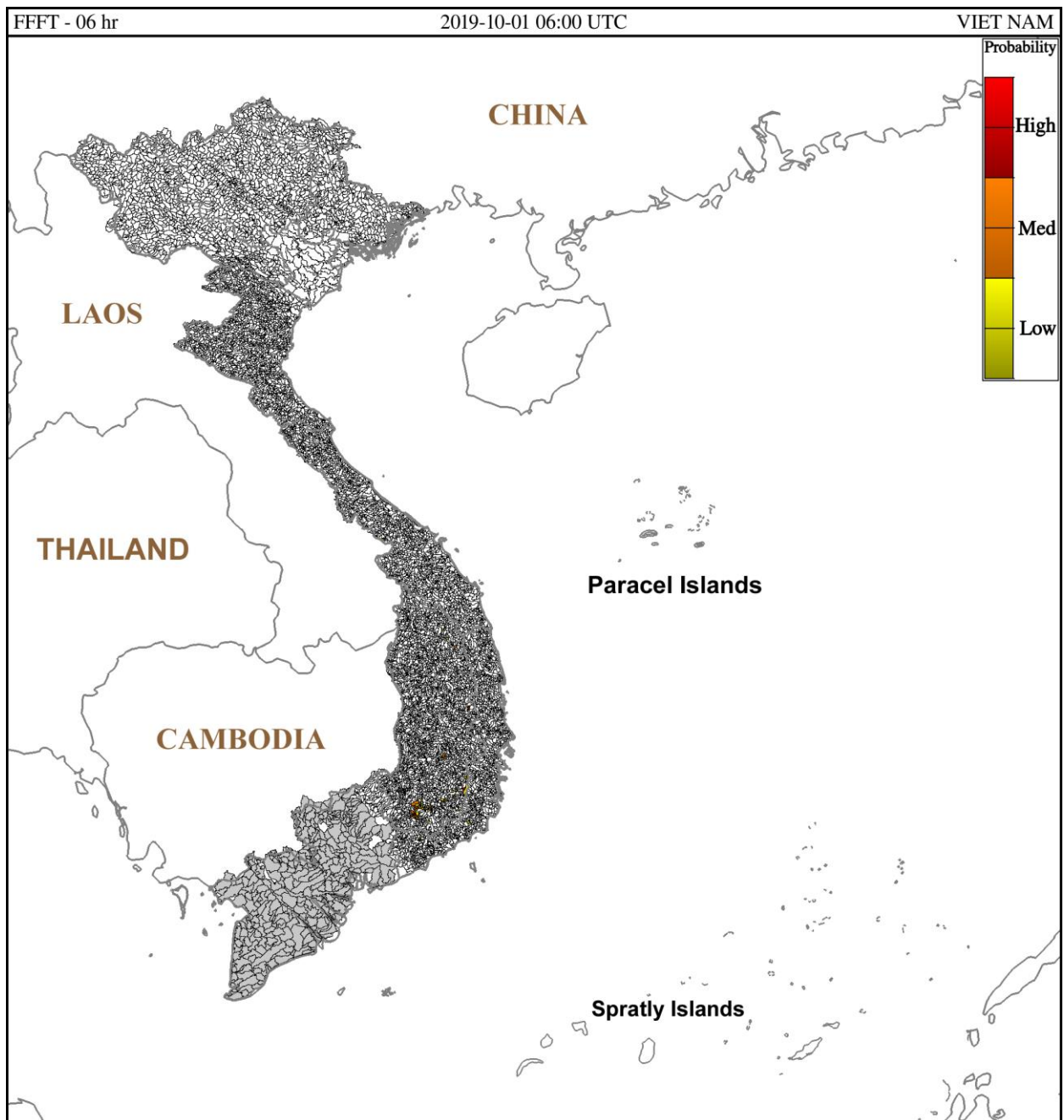
Hình 1: Nguy cơ lũ quét trong 6 giờ tới tại các lưu vực từ 13h ngày 01/10/2019 giờ địa phương
