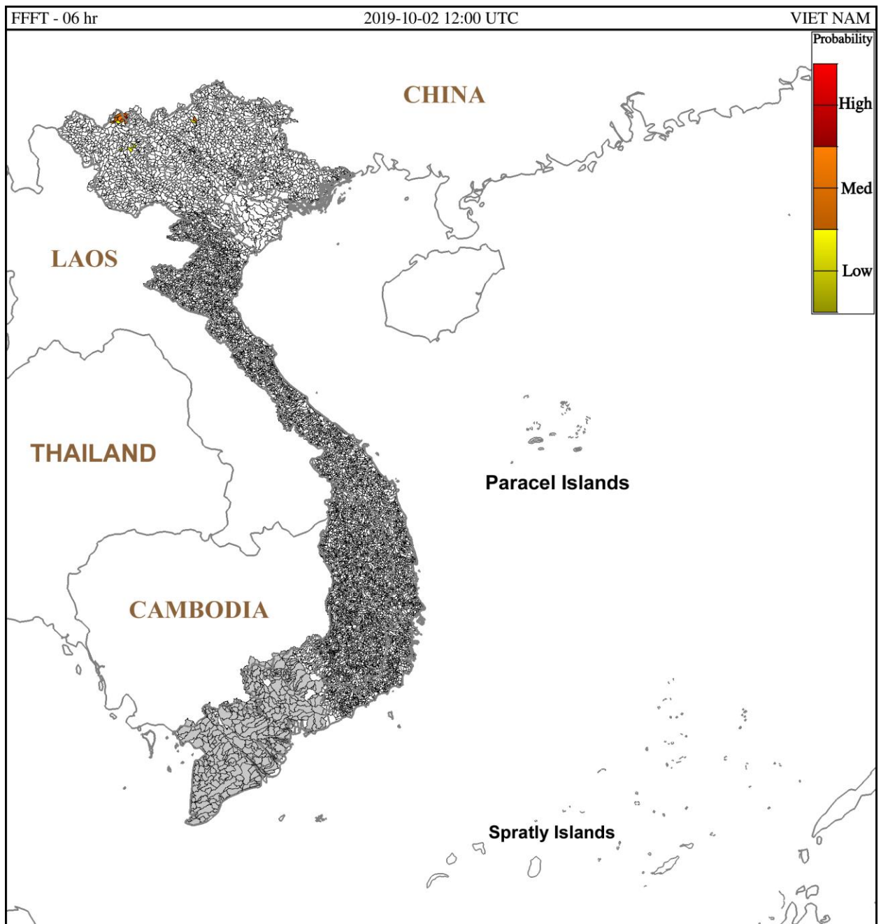
Hình 1: Nguy cơ lũ quét trong 6 giờ tới tại các lưu vực từ 19h ngày 02/10/2019 giờ địa phương
