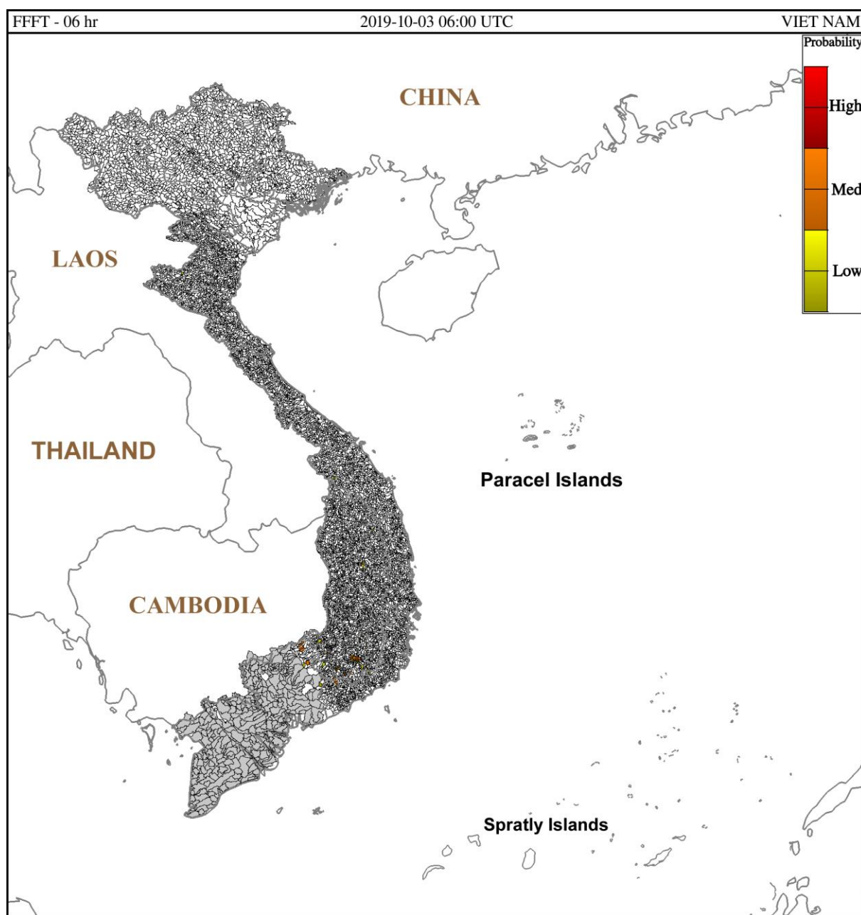
Hình 1: Nguy cơ lũ quét trong 6 giờ tới tại các lưu vực từ 13h ngày 03/10/2019 giờ địa phương
