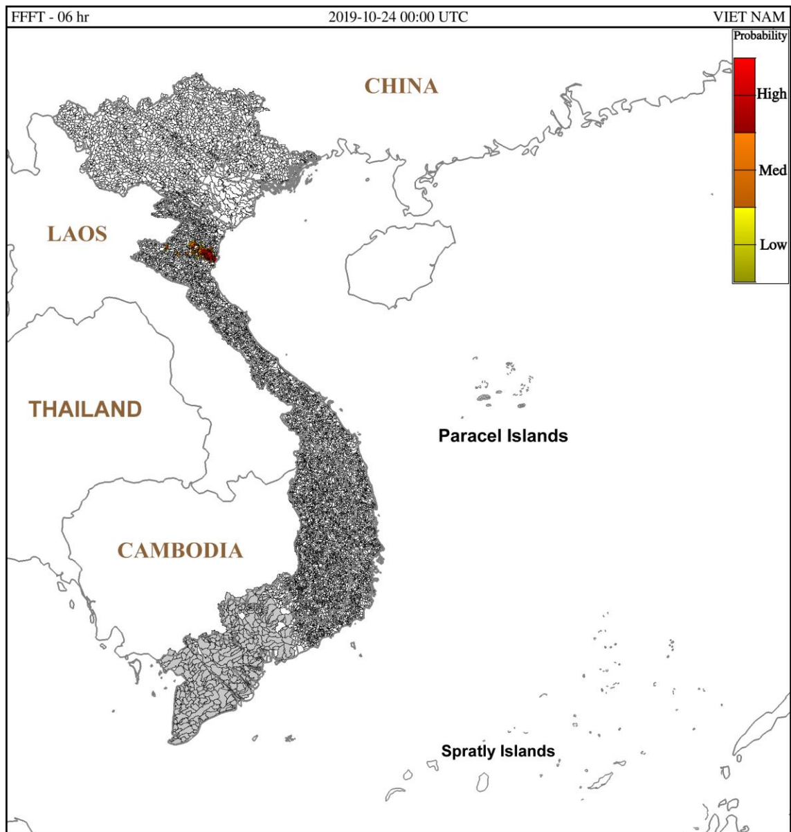
Hình 1. Nguy cơ lũ quét trong 6 giờ tới tại các lưu vực từ 07h ngày 24/10/2019 giờ địa phương
