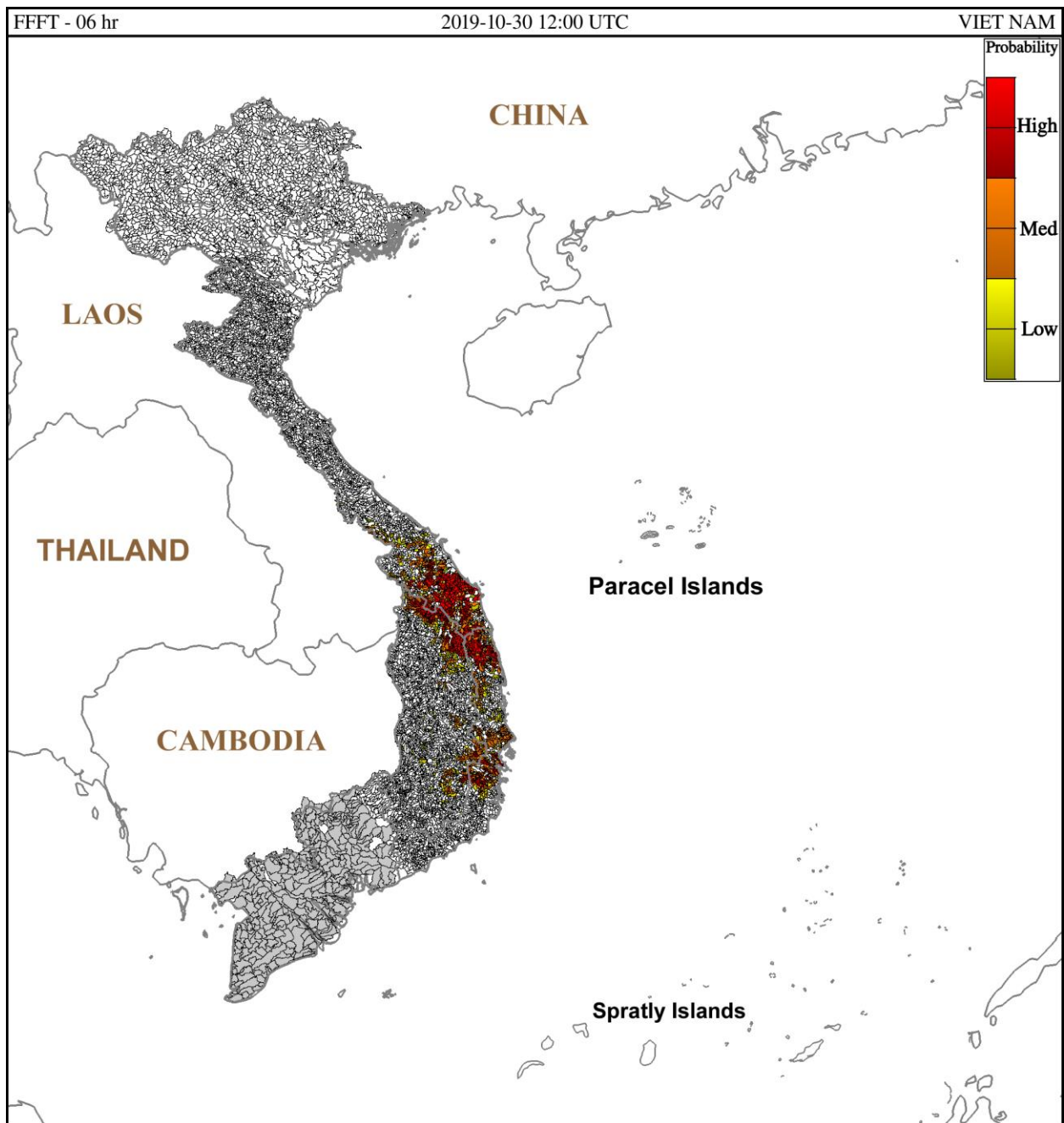
Hình 1: Nguy cơ lũ quét trong 6 giờ tới tại các lưu vực từ 19h ngày 30/10/2019 giờ địa phương
