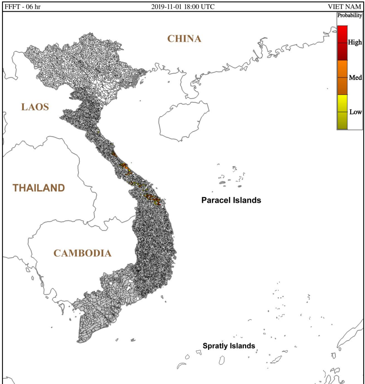
Hình 1. Nguy cơ lũ quét trong 6 giờ tới tại các lưu vực từ 01h ngày 02/11/2019 giờ địa phương
