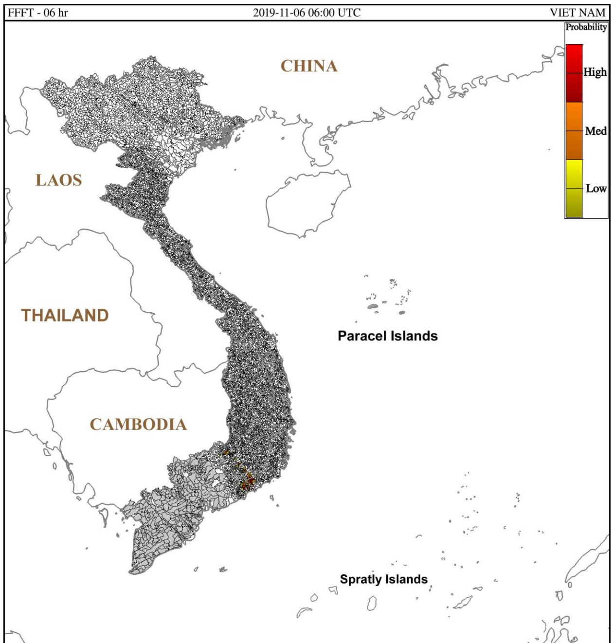
Hình 1: Nguy cơ lũ quét trong 6 giờ tới tại các lưu vực từ 13h ngày 06/11/2019 giờ địa phương
