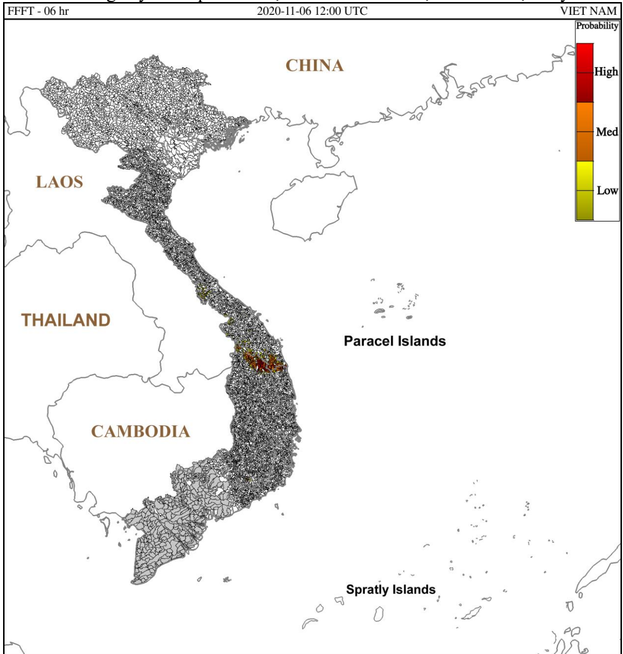
Hình 1. Nguy cơ lũ quét trong 6 giờ tới tại các lưu vực từ 19h ngày 06/11/2020 giờ địa phương
