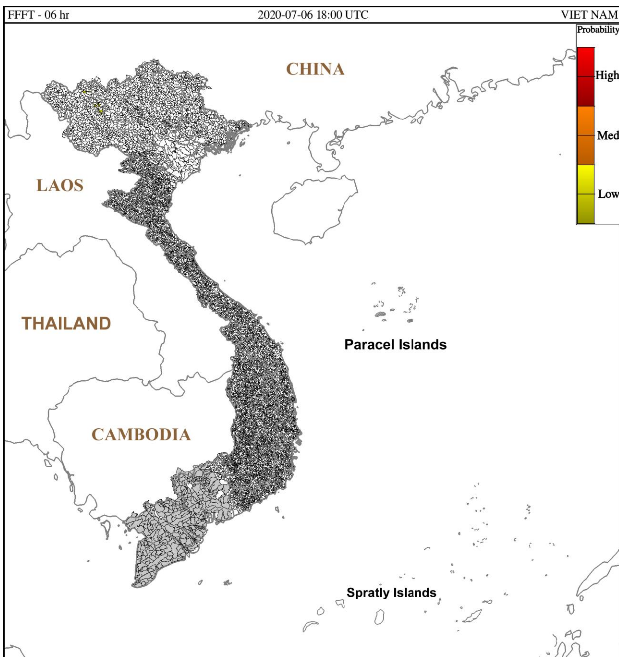
Hình 1. Nguy cơ lũ quét trong 6 giờ tới tại các lưu vực từ 01h ngày 07/07/2020 giờ địa phương
