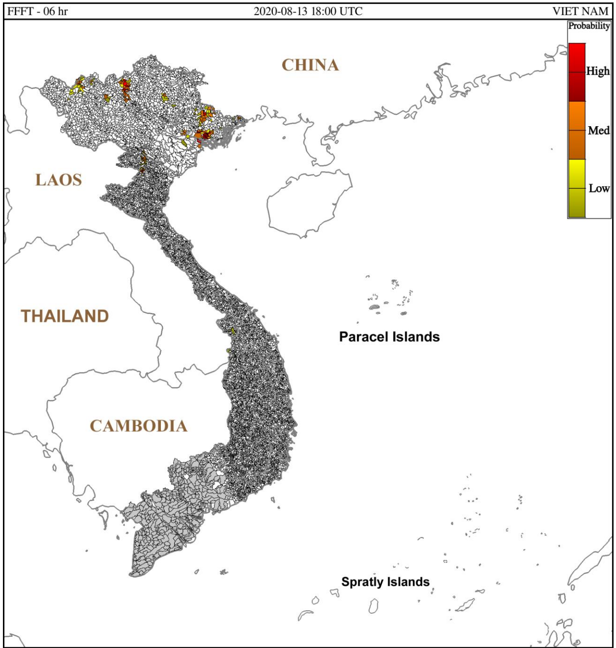
Hình 1: Nguy cơ lũ quét trong 6 giờ tới tại các khu vực từ 01h ngày 14/08/2020 giờ địa phương
