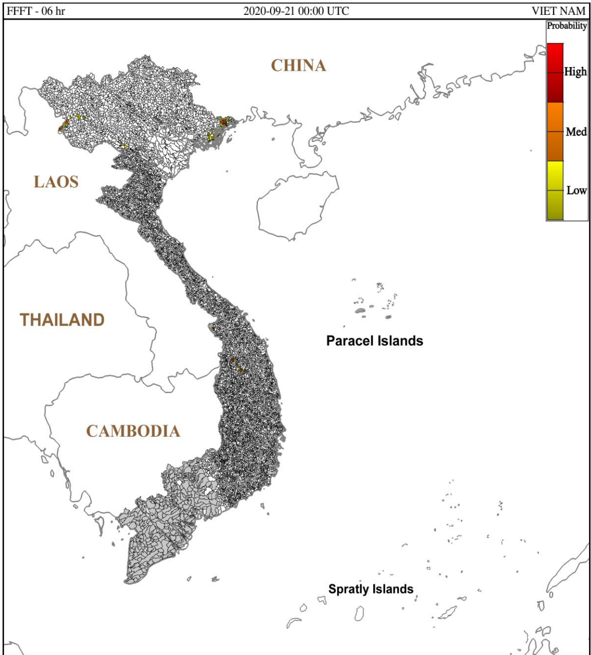
Hình 1: Nguy cơ lũ quét trong 6 giờ tới tại các khu vực từ 07h ngày 21/09/2020 giờ địa phương
