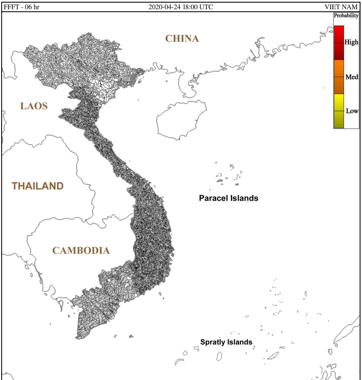
Hình 1. Nguy cơ lũ quét trong 6 giờ tới tại các lưu vực từ 01h ngày 25/04/2020 giờ địa phương
