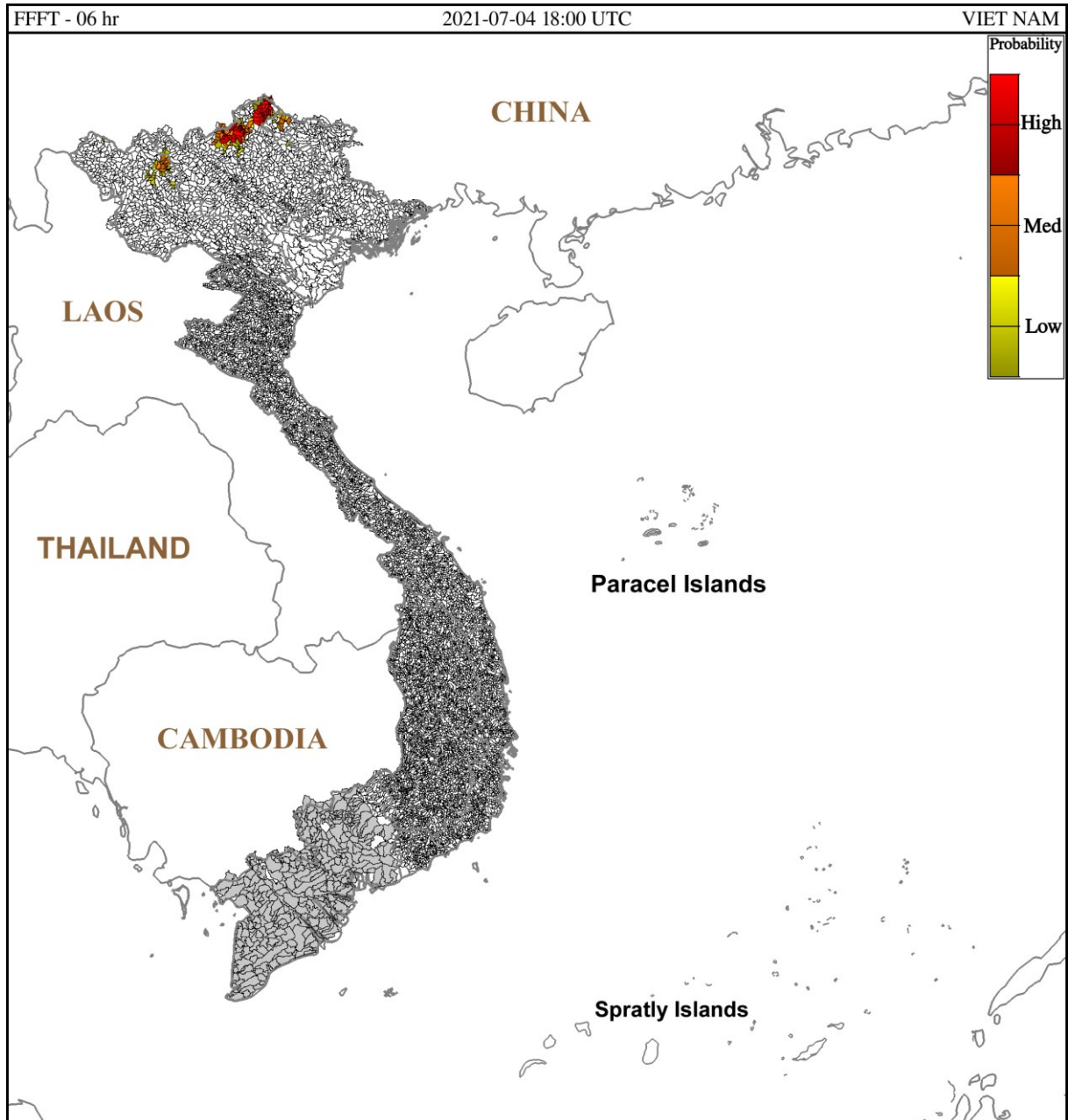
Hình 1. Nguy cơ lũ quét trong 6 giờ tới tại các lưu vực từ 01h ngày 05/07/2021 giờ địa phương
