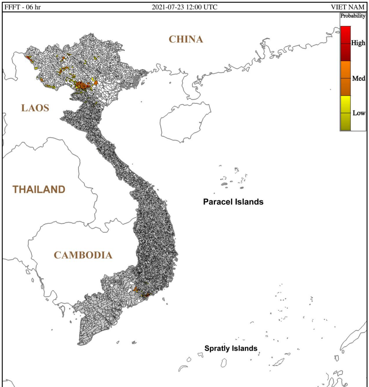
Hình 1. Nguy cơ lũ quét trong 6 giờ tới tại các lưu vực từ 19h ngày 23/07/2021 giờ địa phương
