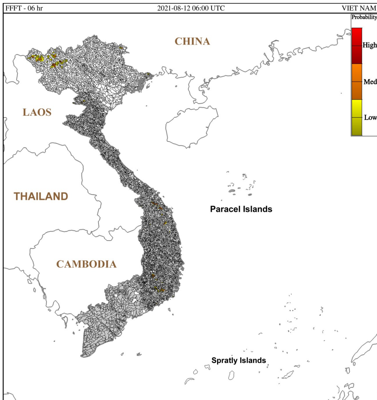
Hình 1. Nguy cơ lũ quét trong 6 giờ tới tại các lưu vực từ 13h ngày 12/08/2021 giờ địa phương
