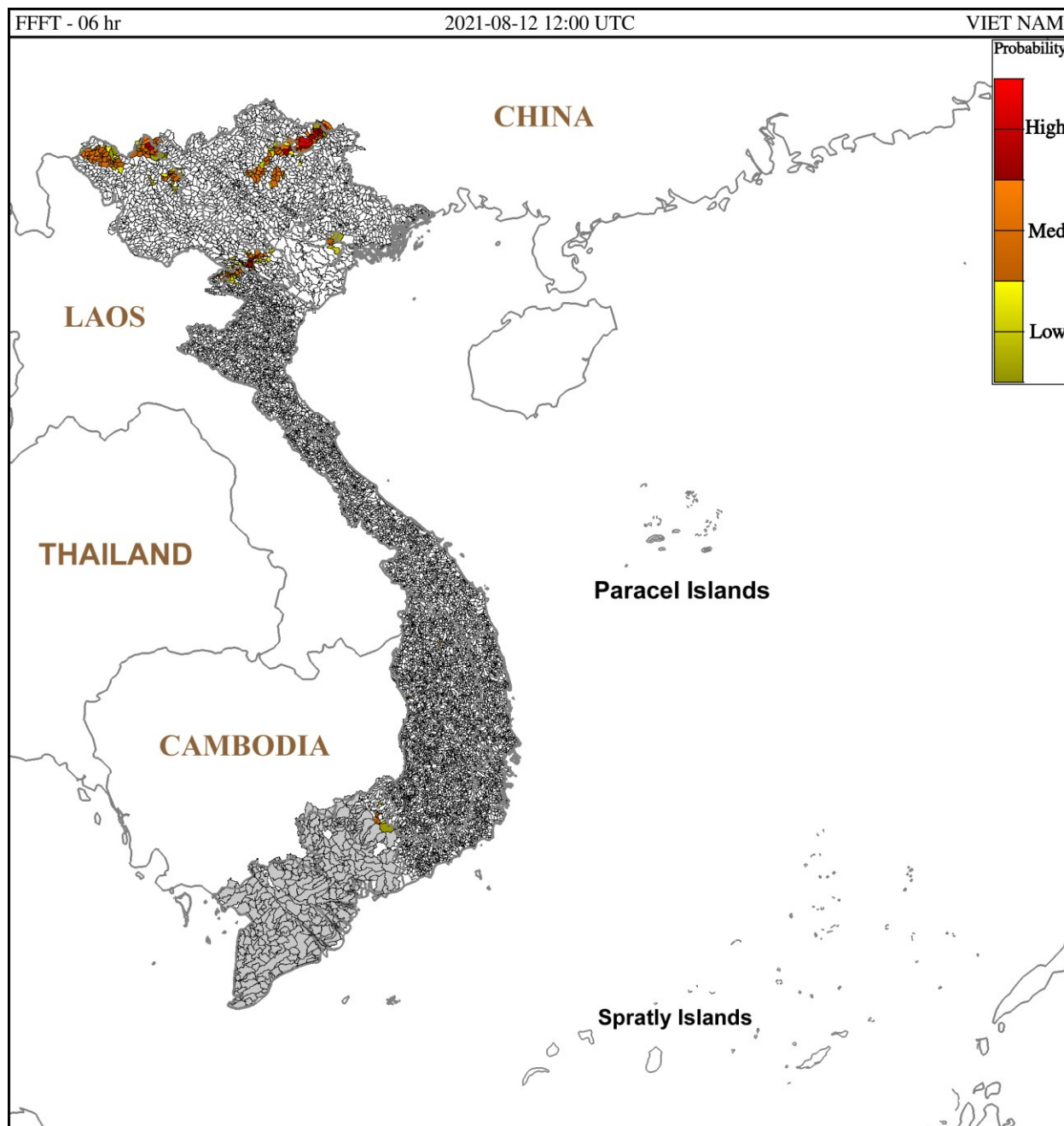
Hình 1. Nguy cơ lũ quét trong 6 giờ tới tại các lưu vực từ 19h ngày 12/08/2021 giờ địa phương
