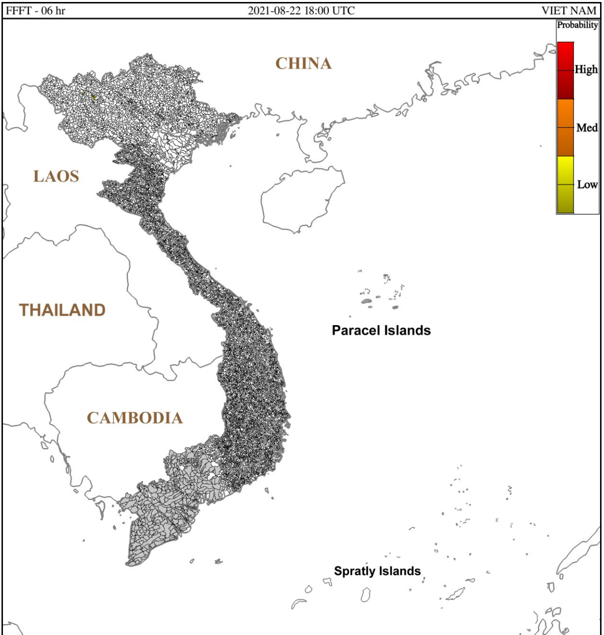
Hình 1. Nguy cơ lũ quét trong 6 giờ tới tại các lưu vực từ 1h ngày 23/8/2021 giờ địa phương
