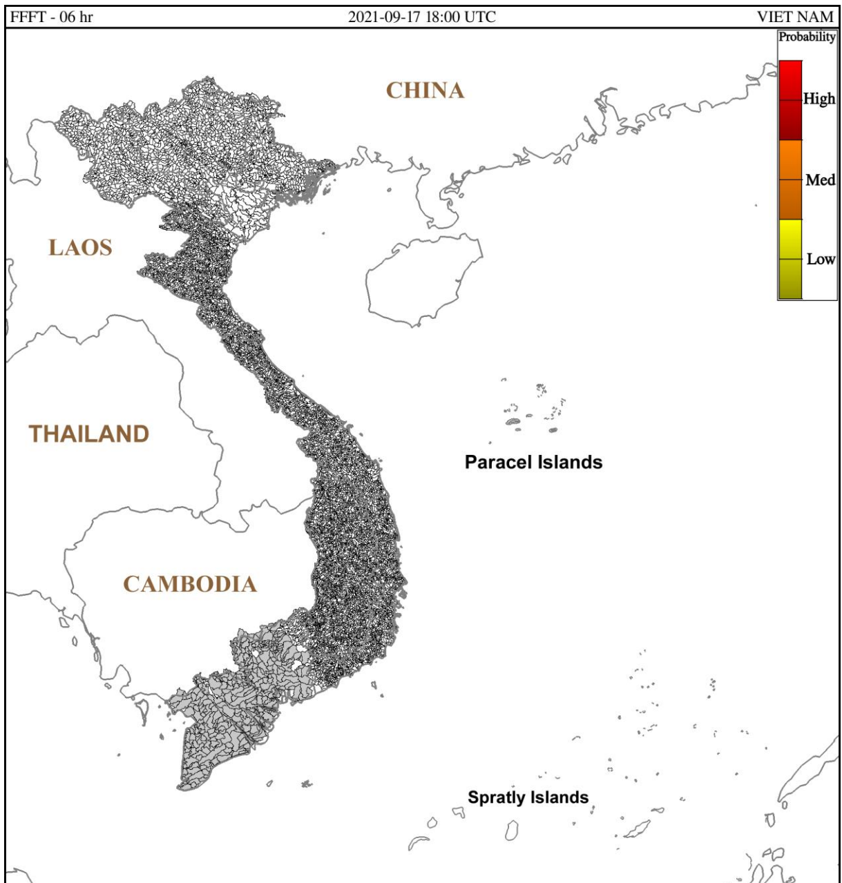
Hình 1. Nguy cơ lũ quét trong 6 giờ tới tại các lưu vực từ 01h ngày 18/09/2021 giờ địa phương
