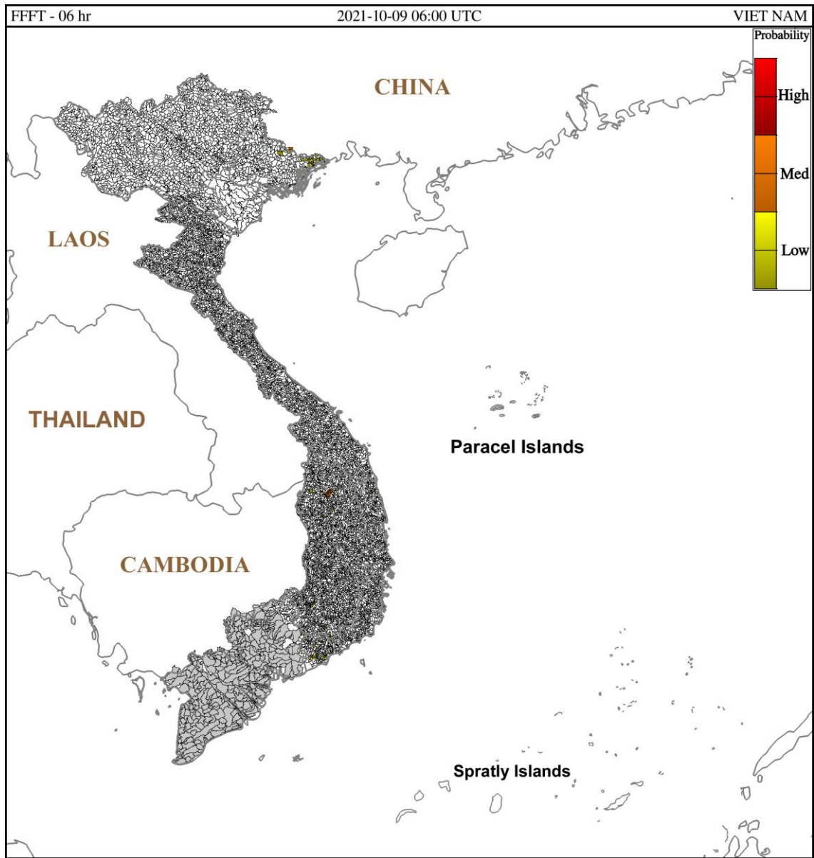
Hình 1. Nguy cơ lũ quét trong 6 giờ tới tại các lưu vực từ 13h ngày 09/10/2021 giờ địa phương
