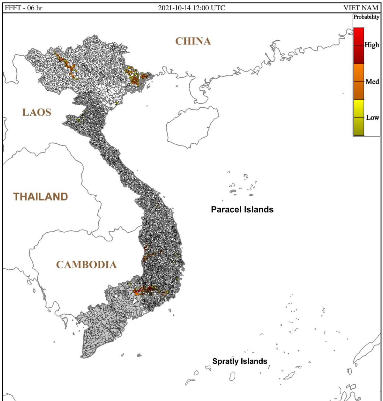
Hình 1. Nguy cơ lũ quét trong 6 giờ tới tại các lưu vực từ 19h ngày 14/10/2021 giờ địa phương
