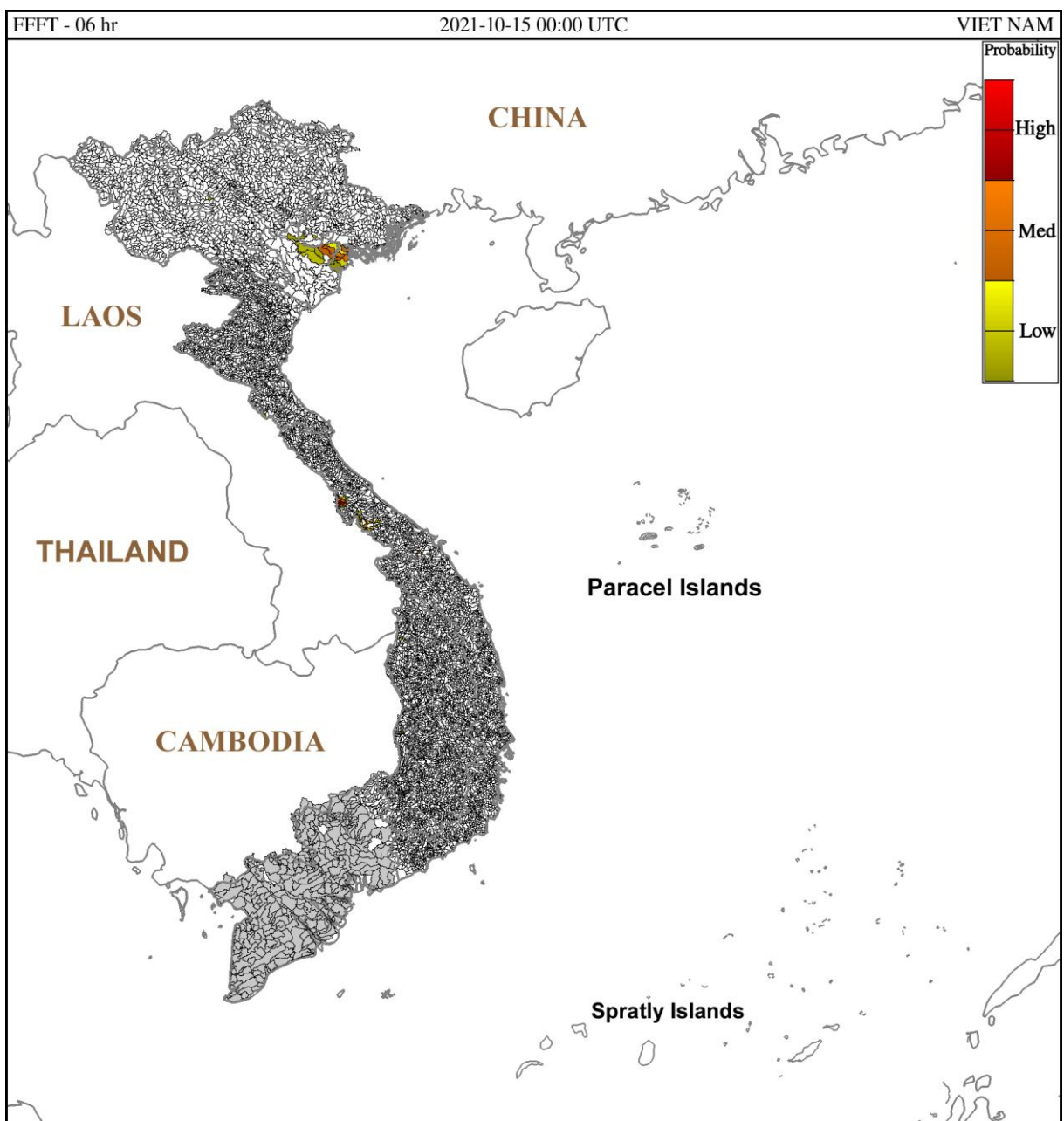
Hình 1. Nguy cơ lũ quét trong 6 giờ tới tại các lưu vực từ 07h ngày 15/10/2021 giờ địa phương
