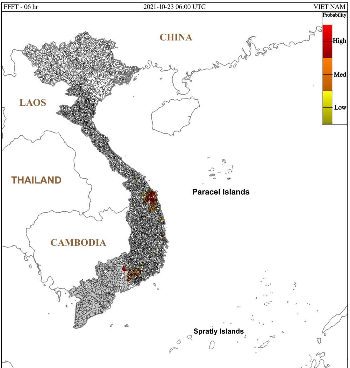
Hình 1. Nguy cơ lũ quét trong 6 giờ tới tại các lưu vực từ 13h ngày 23/10/2021 giờ địa phương
