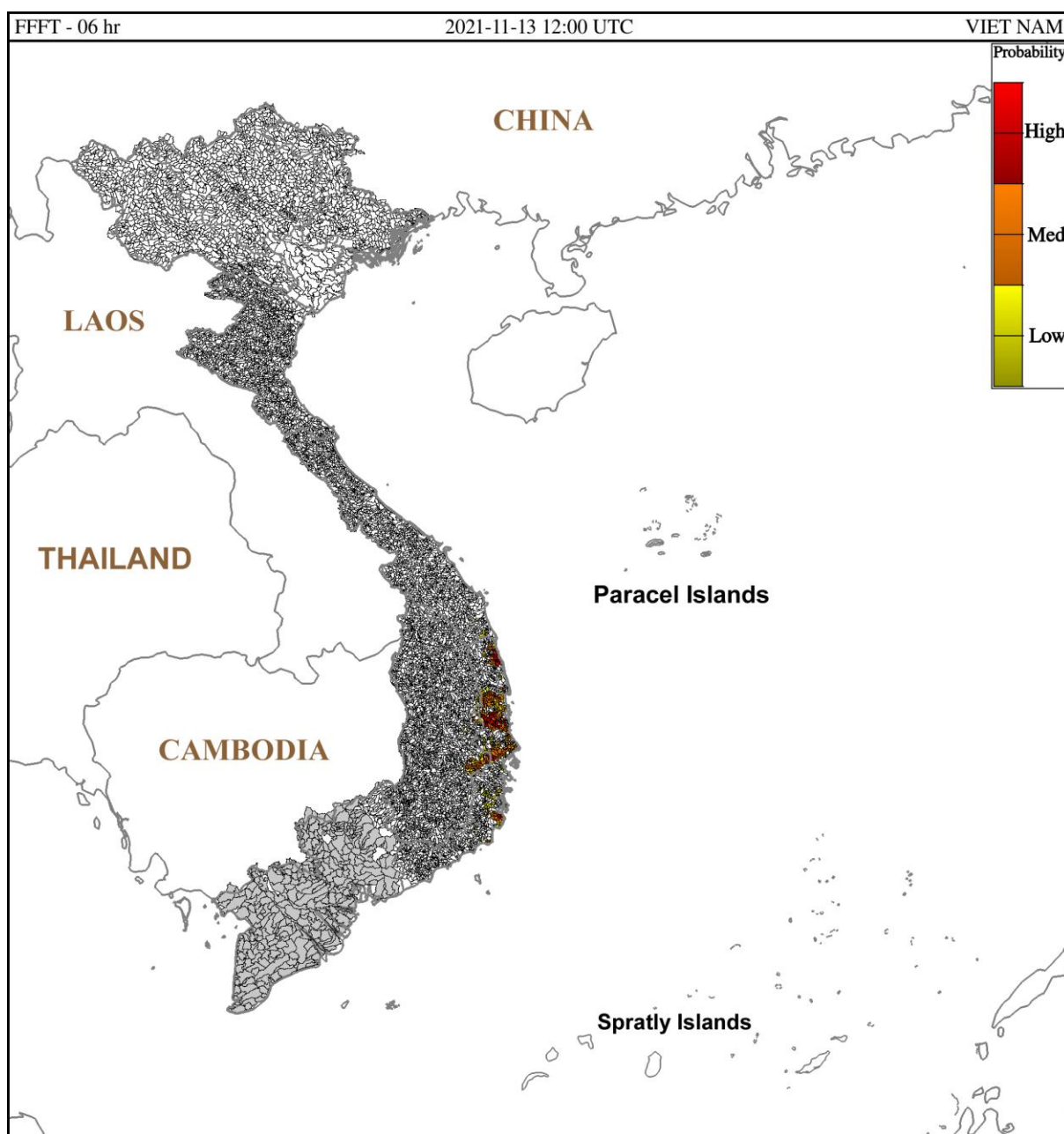
Hình 1. Nguy cơ lũ quét trong 6 giờ tới tại các lưu vực từ 19h ngày 13/11/2021 giờ địa phương
