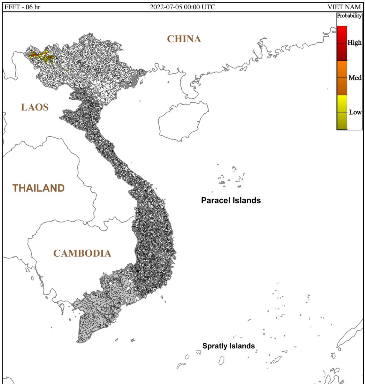
Hình 1. Nguy cơ lũ quét trong 6 giờ tới tại các lưu vực từ 07h ngày 05/07/2022 giờ địa phương
