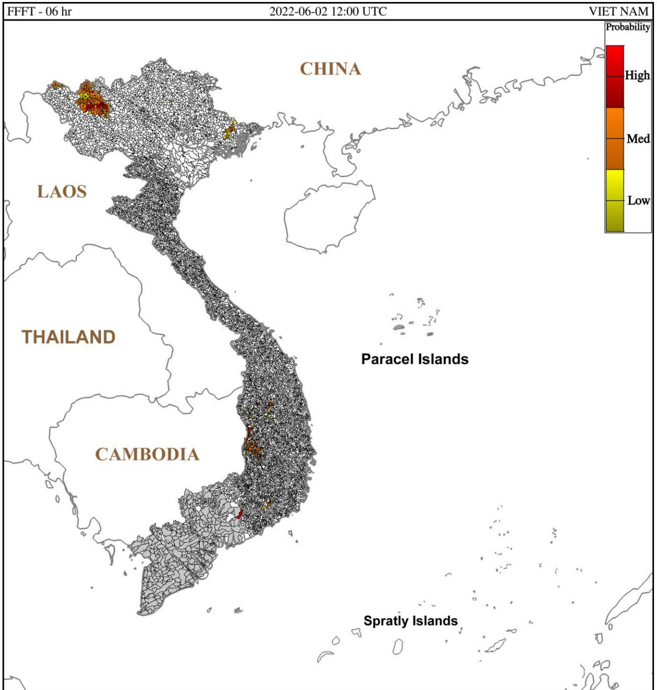
Hình 1: Nguy cơ lũ quét trong 6 giờ tới tại các lưu vực từ 19h ngày 02/6/2022 giờ địa phương
