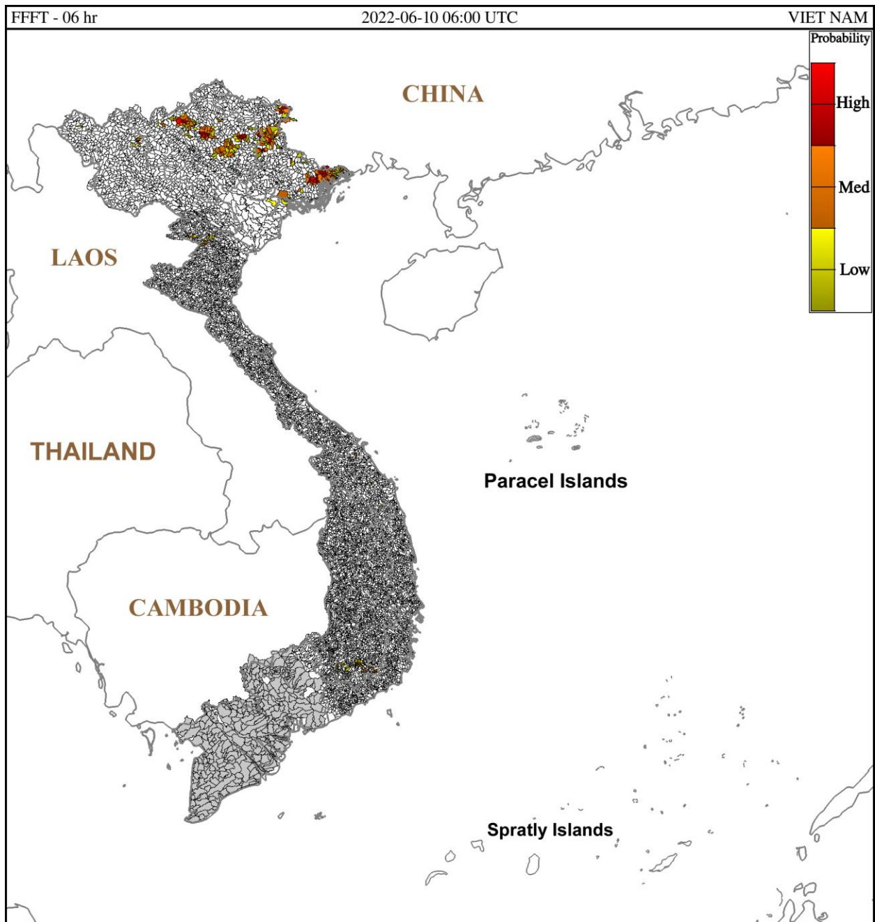
Hình 1. Nguy cơ lũ quét trong 6 giờ tới tại các lưu vực từ 13h ngày 10/06/2022 giờ địa phương
